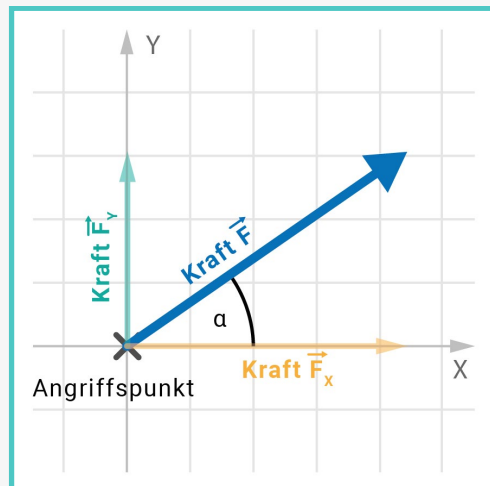
Abb.: Kraft und die Kraftkomponenten in x- und y-Richtung.
