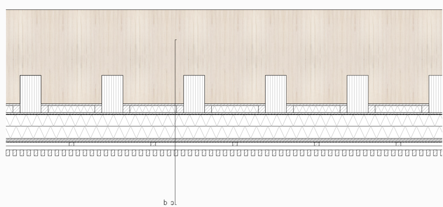
FASSADENSCHNITT a-a HORIZONTAL HAUPTHAUS M120
