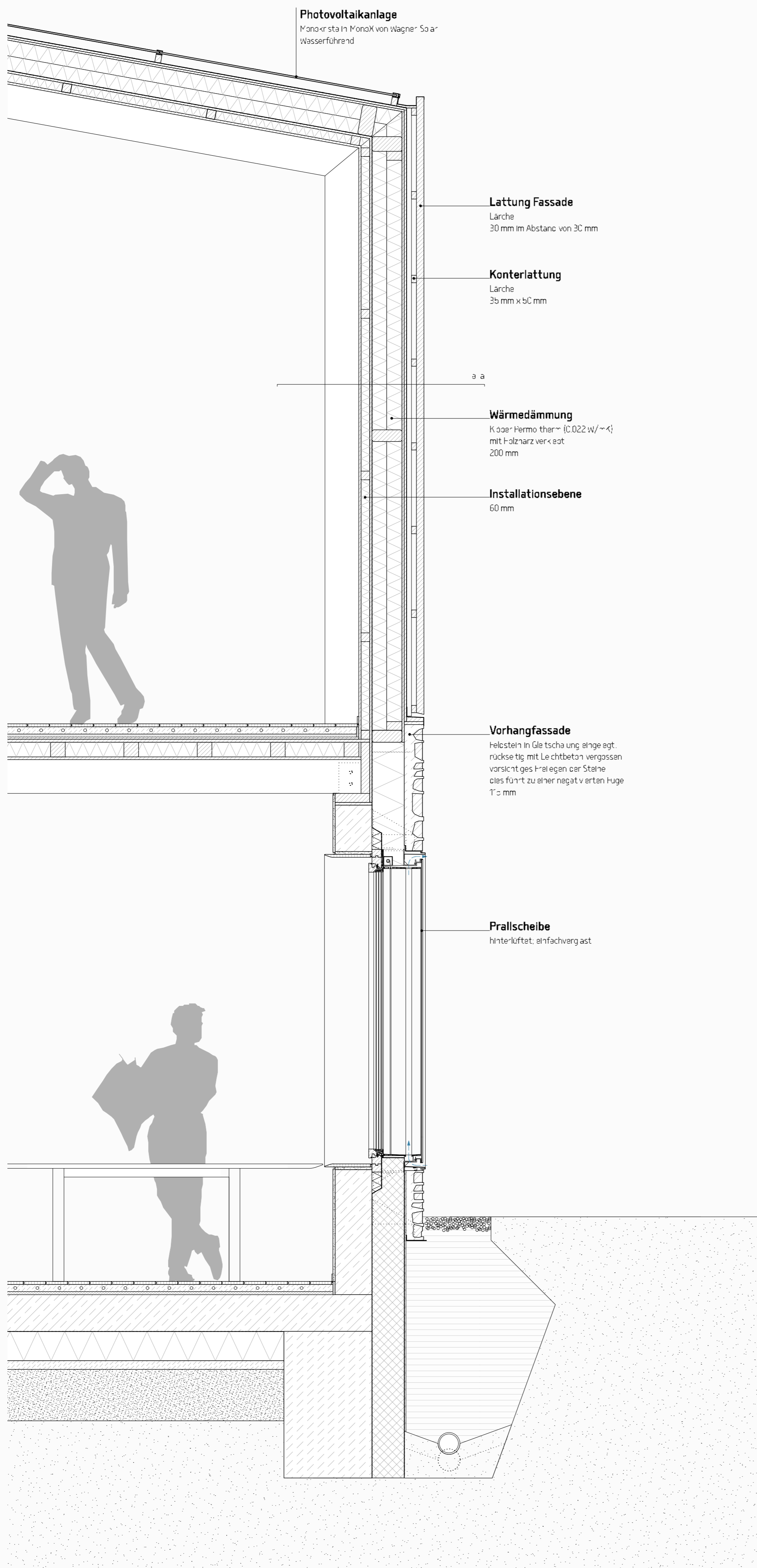
FASSADENSCHNITT b-b HAUPTHAUS M120
