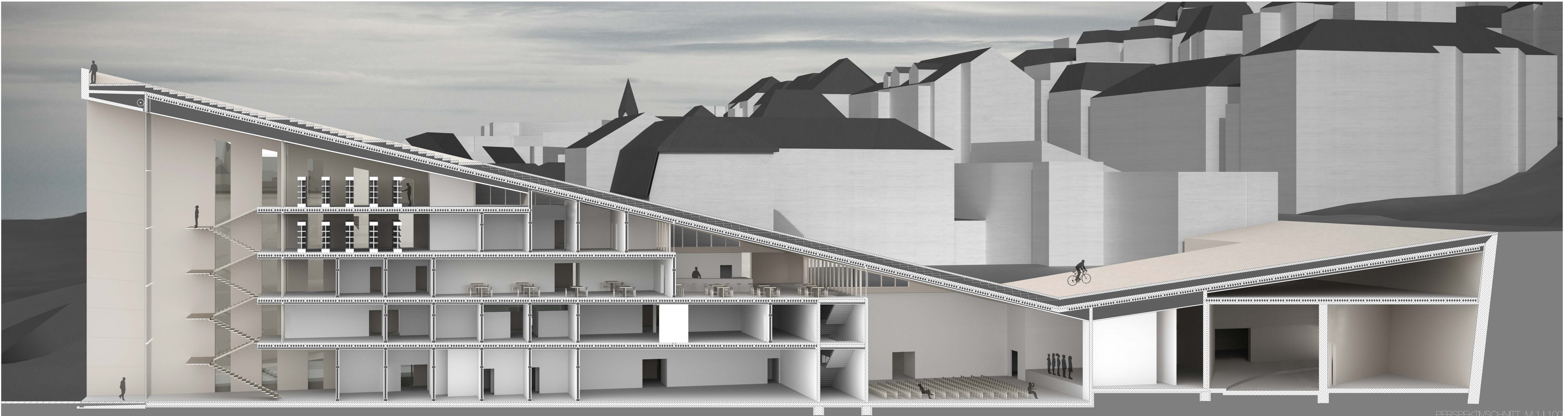
PERSPEKTIVSCHNITT M 1:1 100 BT BAT QUIN DILLING
