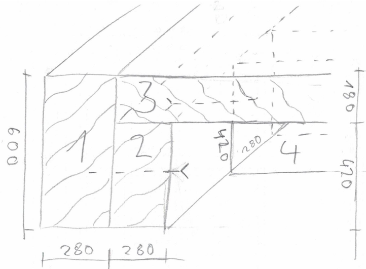
Aussteifung mit Beinen und Unterkonstruktion verschraubt
