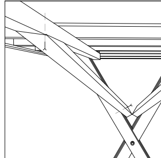
Aussteifung mit Beinen und Unterkonstruktion verschraubt
