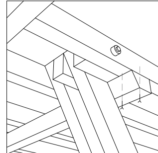
Verschraubung der Bretter(Tischplatte) auf Unterkonstruktion
