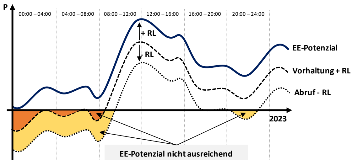
Abbildung 13: Schematisches Regelleistungspotenzial – Wind
