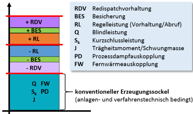
Abbildung 2: Konventioneller Erzeugungssockel
