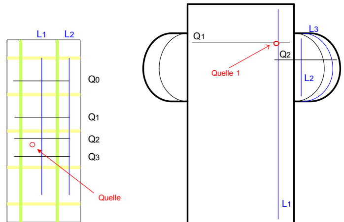
Abb. 1: Verrippte Platte (links), Bodenblech (rechts) mit Radhäusern und Randdämpfung (dick)
