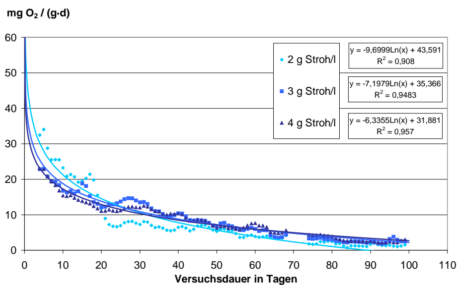
Abbildung 3.18 Zeitliche Entwicklung des Sauerstoffumsatzes in \text{mg O}_2/(\text{g Stroh} \cdot \text{d}) bei geringer Substrateinwaage
