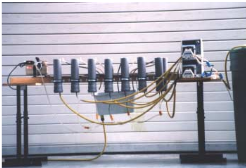
Abbildung 4.3 Säulenversuchsanlage zur Adsorption von Phosphaten
