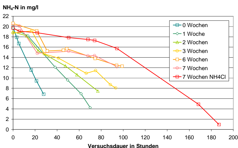
Abbildung 3.2 Abnahme der Ammoniumkonzentration nach Mangelphasen von bis zu 7 Wochen
