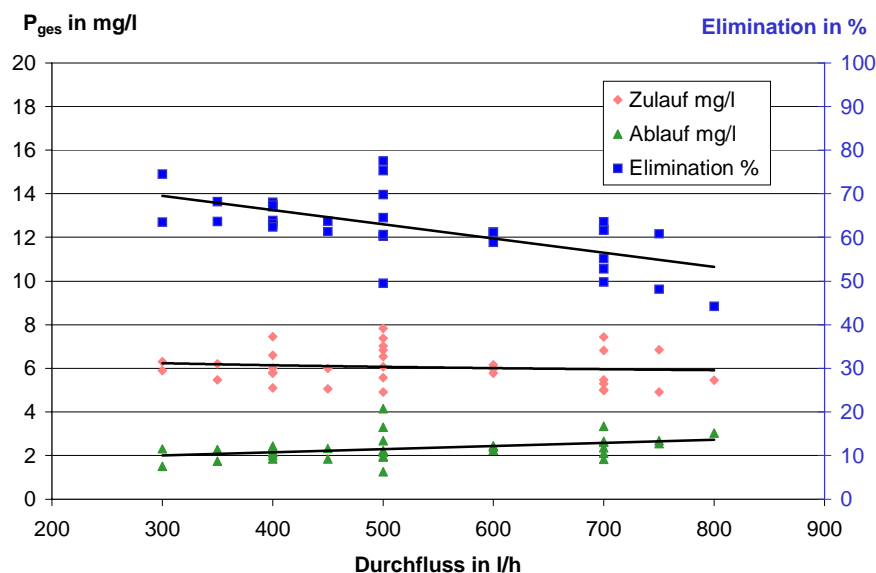
Abbildung 4.14 Zu- und Ablaufkonzentration sowie Eliminationsrate in Abhängigkeit von der Reaktorbelastung bei täglich mehrmaliger Regeneration
