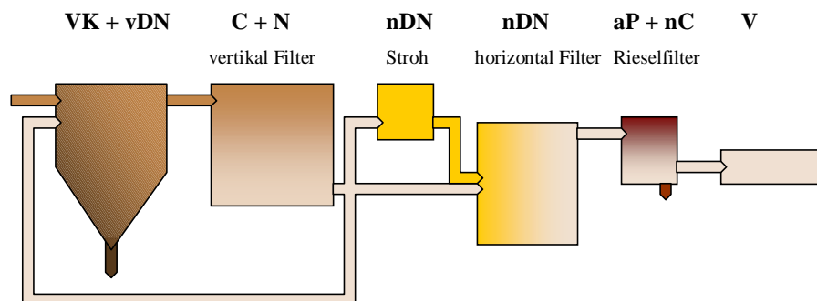
Abbildung 5.3 Verfahrensschema zur weitergehenden Abwasserreinigung mit bewachsenem Bodenfilter als Hauptreinigungsstufe
