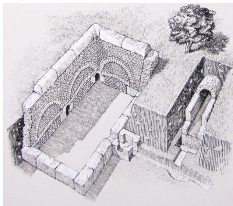
Abbildung 5: a, frei gelegter Abschnitt des römischen Aquädukts bei Obernau, b, Prinzipskizze des römischen Sammelbeckens (Sumelocenna – Römisches Stadtmuseum Rottenburg), c, Reste der römischen Wasserleitung vor dem Stadtmuseum Rottenburg
