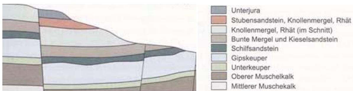
Abb.1: Schematischer geologischer Schnittdurch das Neckartal im Raum Stuttgart (verändert nach Spitzberg und Ufrecht, 2014)
