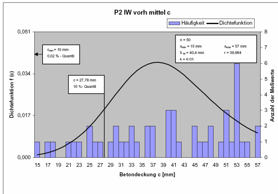
Abb. 51 : Graphische Darstellungen der Häufigkeitsverteilung der vorhandenen mittleren Betondeckung c von 50 Innenwänden der Typenserie P2
