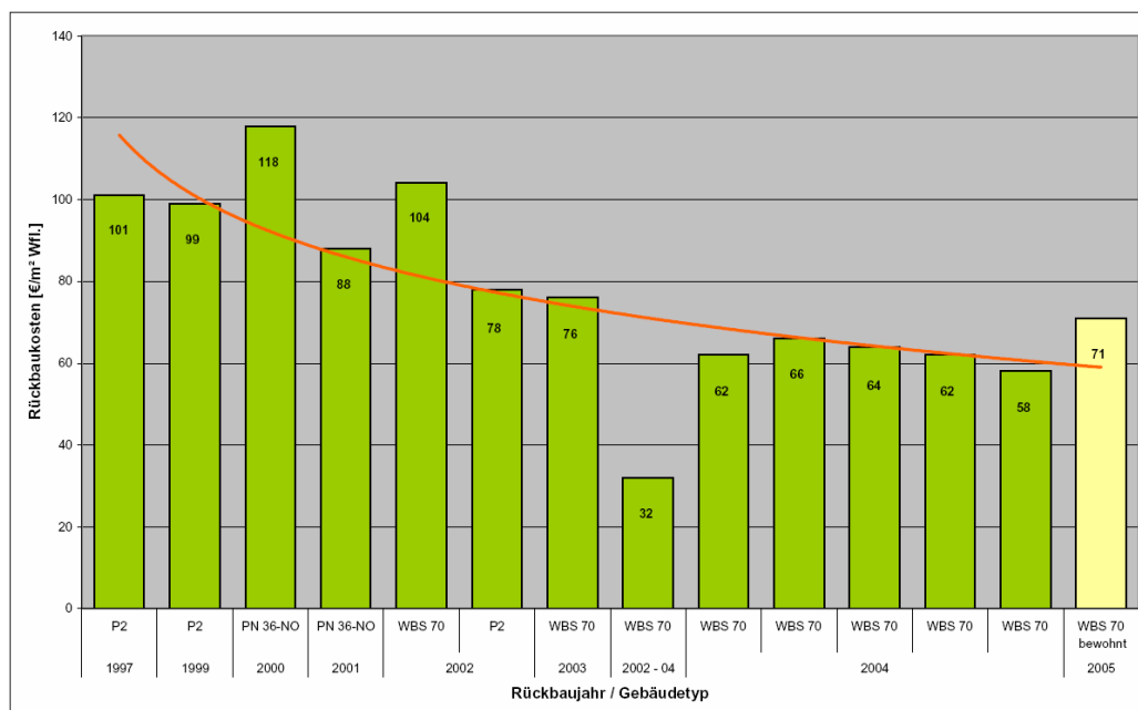
Abb. 99 : Entwicklung der Rückbaukosten
