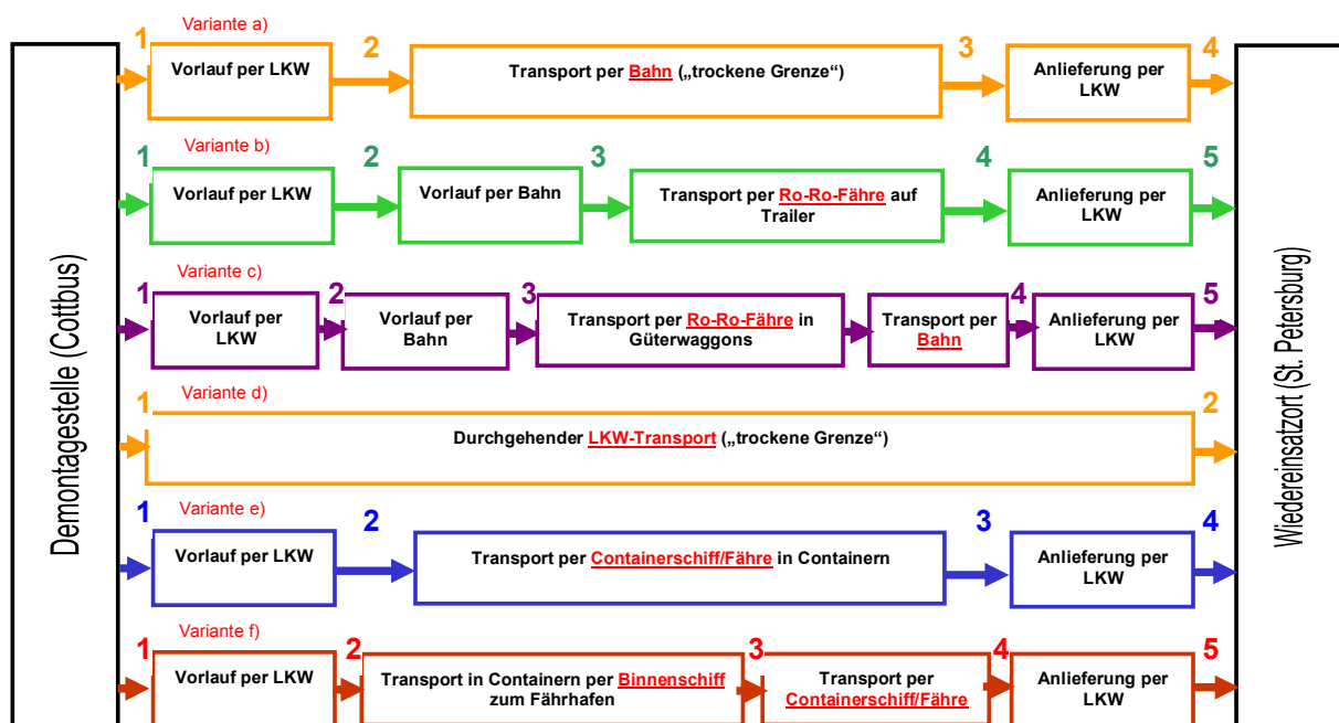
Abb. 101 : Transportwege und –varianten für einen Bauteiltransport nach St. Petersburg 327
