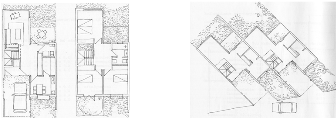
Abb. 150 : Grundrisse der Reihenhaushaus-Konstruktion
