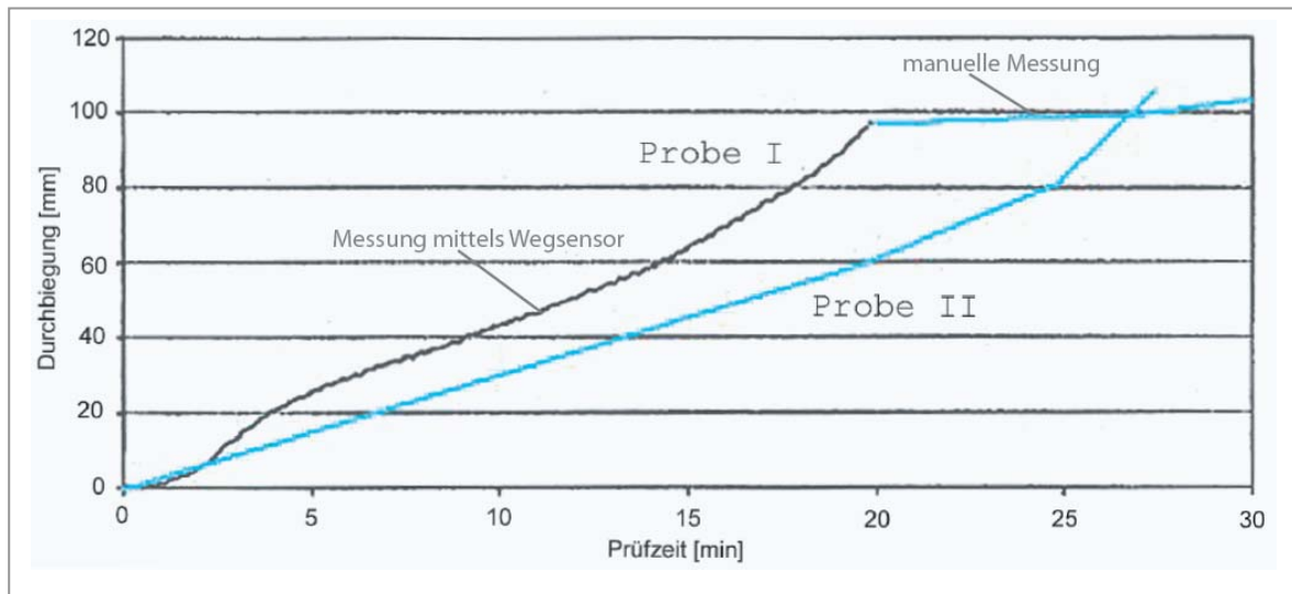
Abb. 74 : Durchbiegung in Richtung Brandraum – Spannbetondeckenplatten 21000 (P2-Typ)
