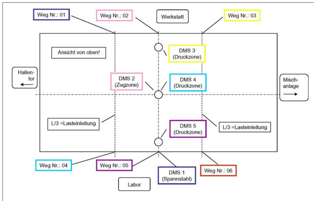
Abb. 55 : Lage der Krafteinleitungslinien und Messstellen zur Untersuchung des Tragverhaltens
