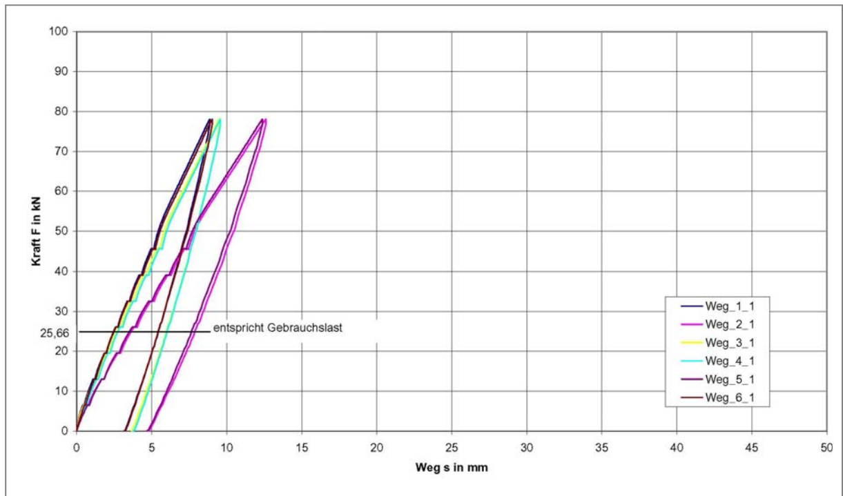
Abb. 62 : Kraft-Weg-Diagramm Stahlbetondecke 2, Elemente-Nr. 21 120
