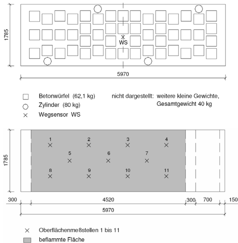
Abb. 70 : Exemplarische Darstellung der Messpunkte und des Belastungsplanes zur Untersuchung des Feuerwiderstandes – Spannbetondeckenplatte 21000
