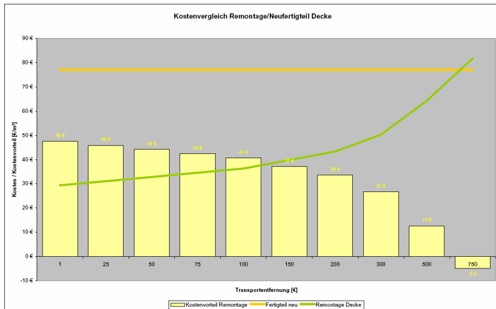
Abb. 117 : Vergleich der Kosten für die Montage von neuen Deckenelementen mit den Remontagekosten sekundärer Bauteile in Abhängigkeit der Transportentfernung (LKW) in Deutschland (beachte. verzerrte Darstellung der Transportentfernung)
