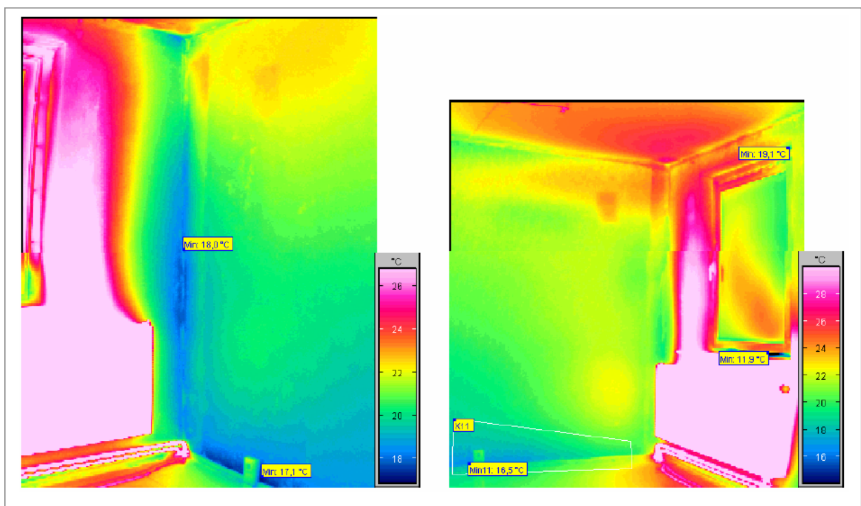
Abb. 69 : Infrarotaufnahmen Außenwanddecke Kinder- (li.) und Wohnzimmer (re.), oberstes Wohngeschoss
