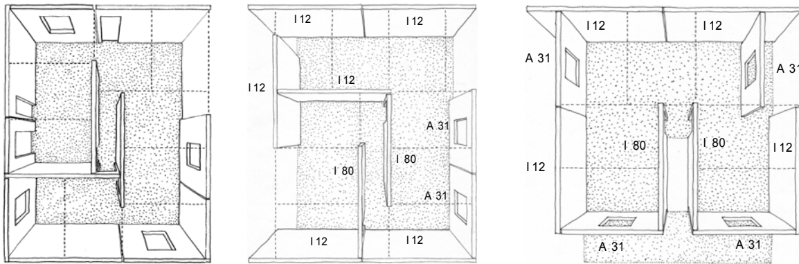
Abb. 146 : Grundrisse der Shell-Haus-Konstruktionen. eingeschossig (li.), zweigeschossig EG (mi.) OG (re.)
