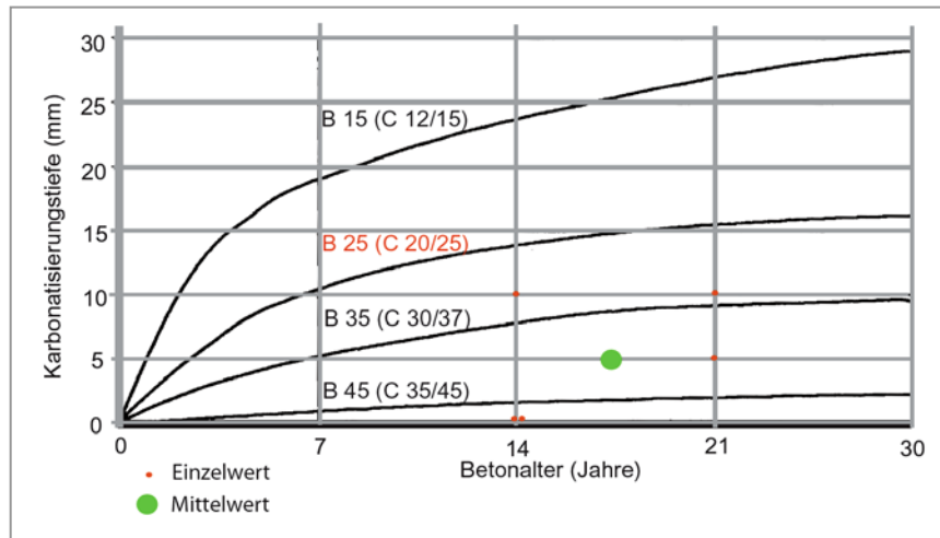
Abb. 42 : Karbonatisierungstiefe der Außenwände des Typs WBS 70
