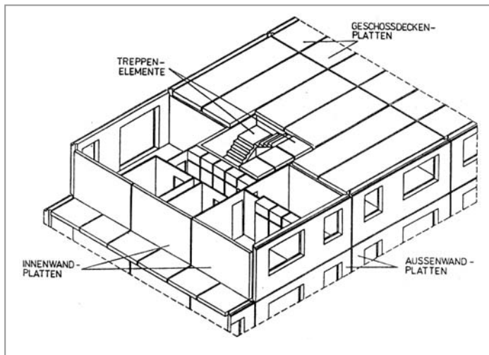
Abb. 19 : Räumliche Darstellung eines P2-Segments 109
