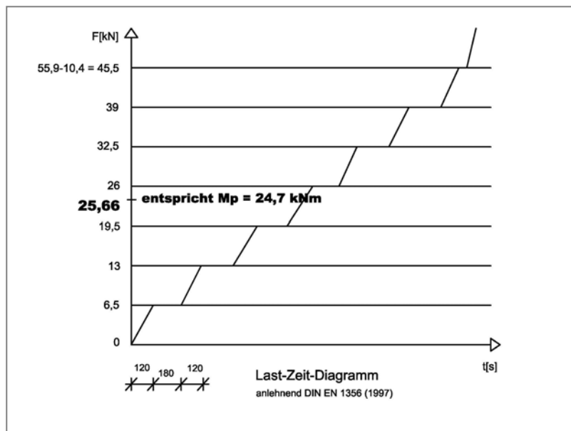
Abb. 61 : Last-Zeit-Diagramm anlehnend an DIN EN 1356: 1997-02
