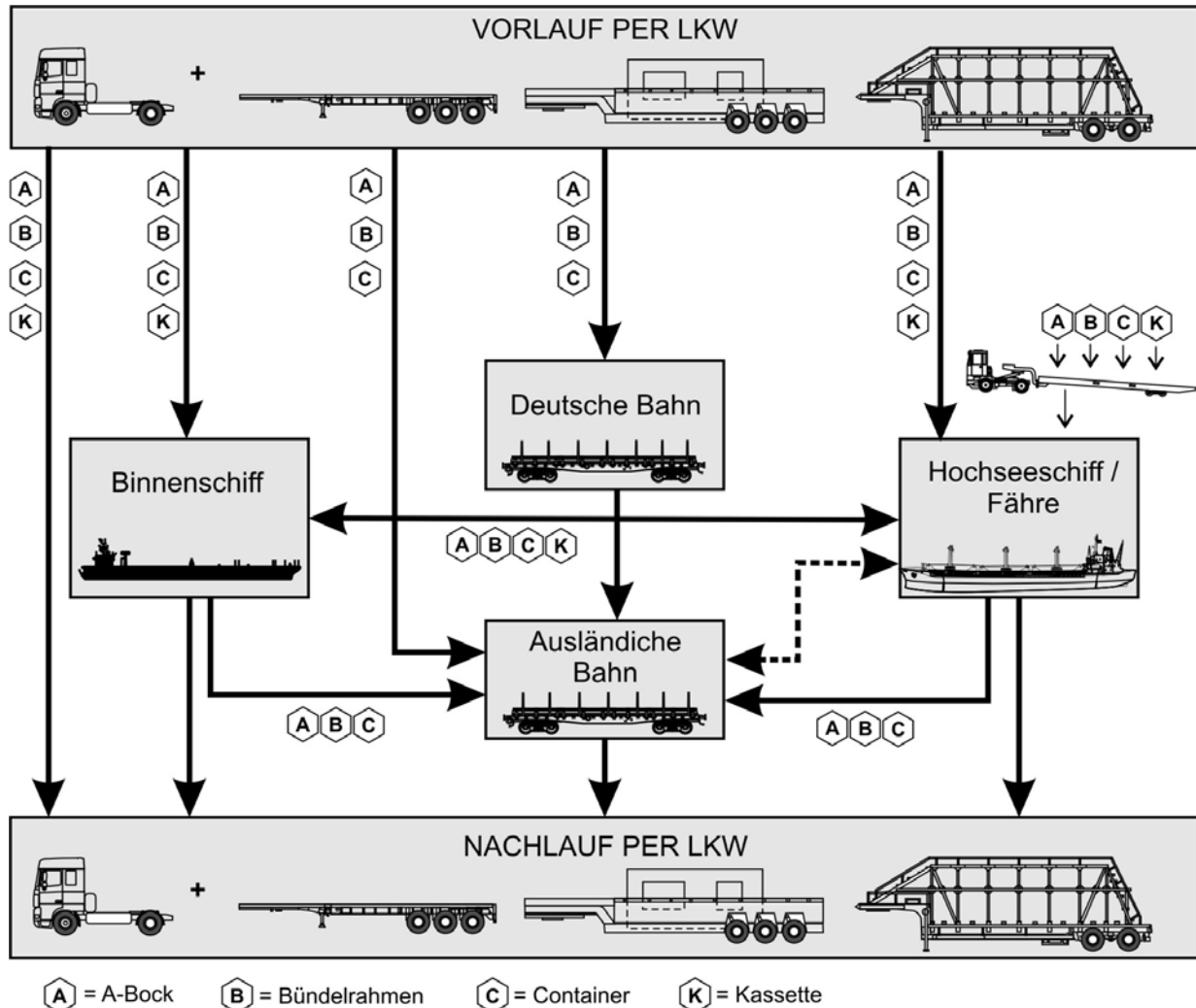
Abb. 93 : Überblick über die geeigneten Kombinationsmöglichkeiten für den Transport gebrauchter Betonfertigteile
