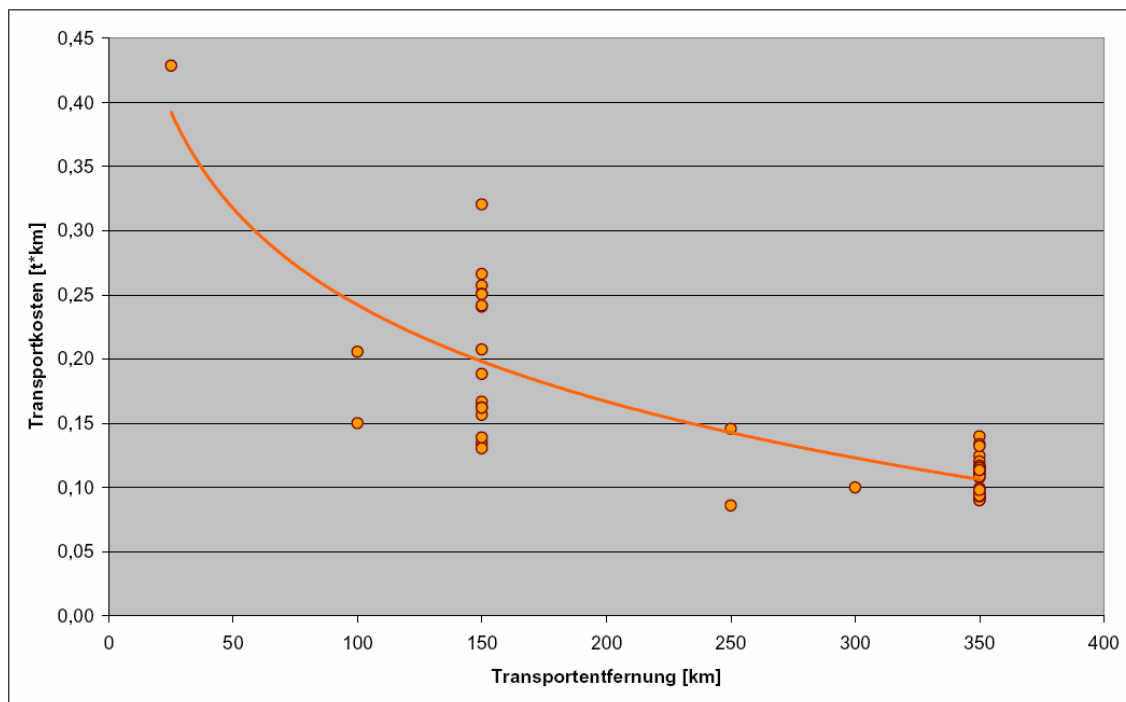
Abb. 103 : Abhängigkeit der LKW-Transportkosten von der Transportentfernung
