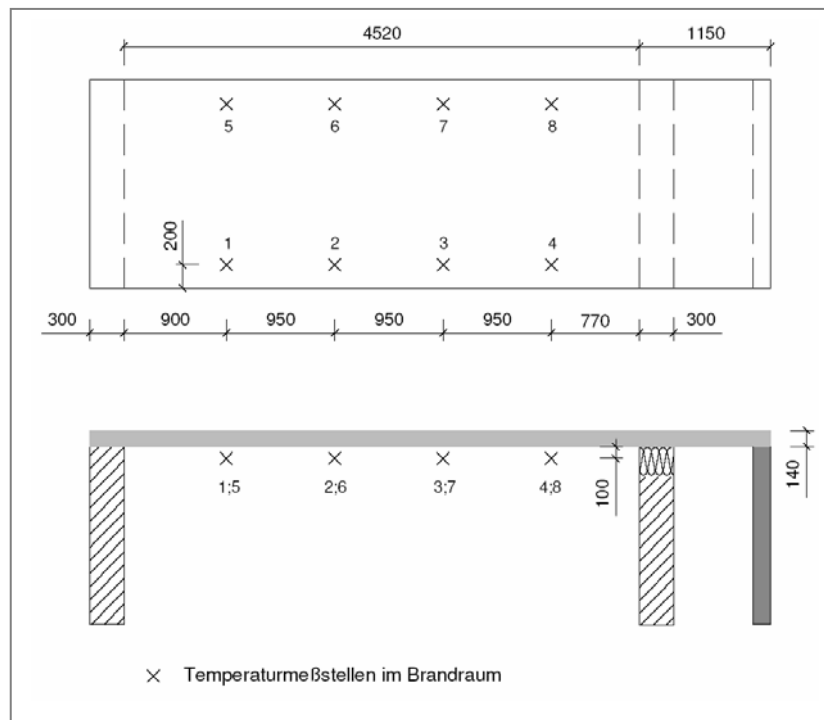
Abb. 72 : Prüfanordnung / Lage der Brandraummessstellen – Spannbetondeckenplatte 21000
