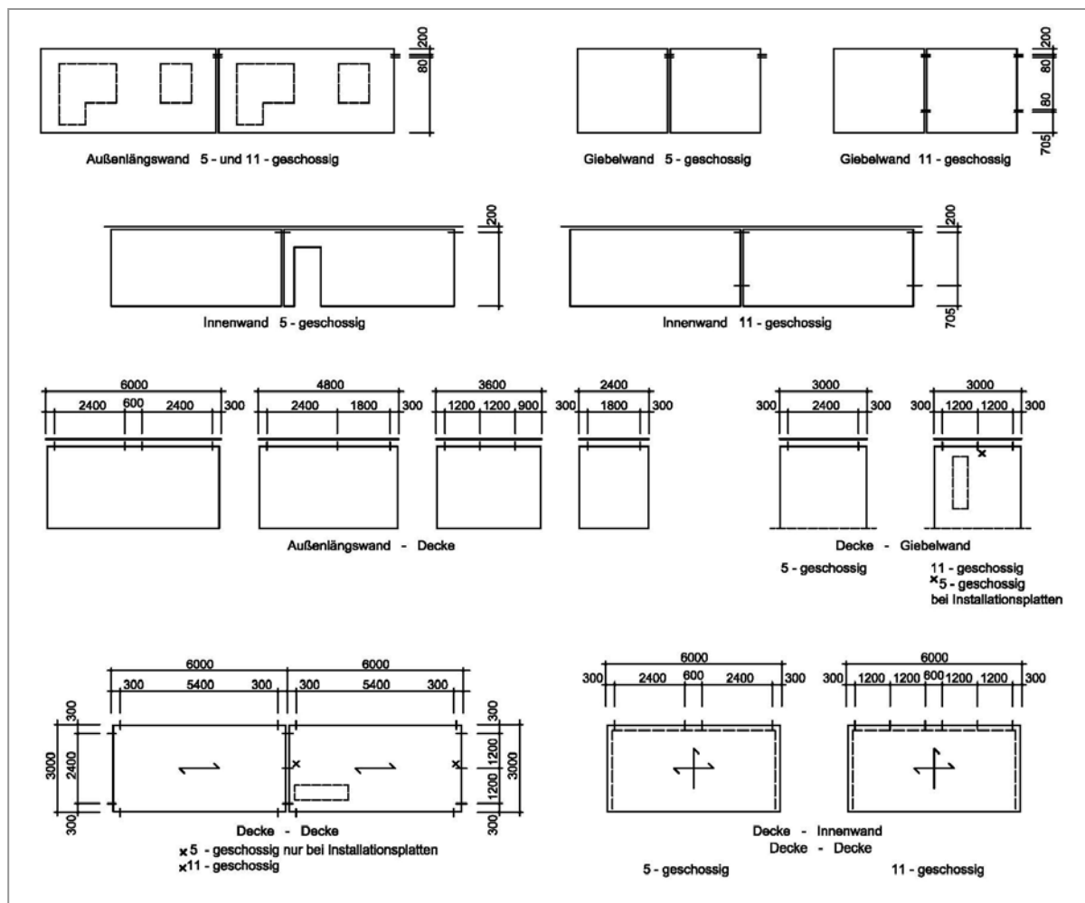
Abb. 32 : Schematische Darstellung der Lage der Schweißverbindungen zwischen den Fertigteilen 154
