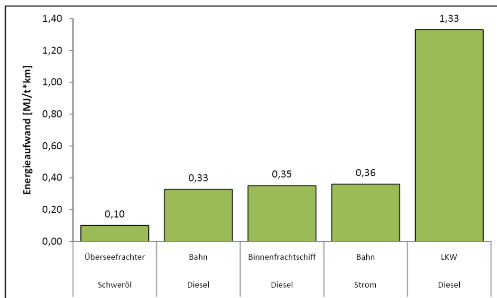
Abb. 129 : Vergleich der Energieaufwendungen für die Demontage und den Abbruch von einer Tonne Betonbauteile
