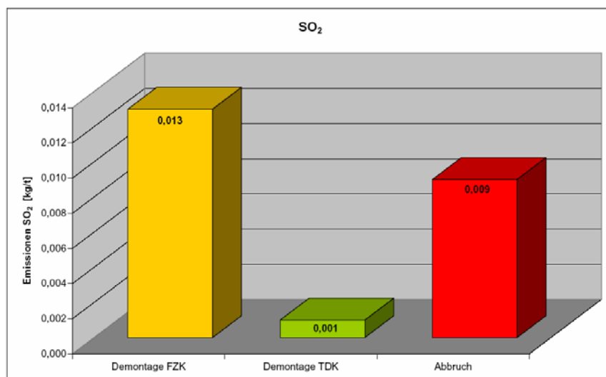
Abb. 132 : Vergleich der \text{SO}_2 -Emissionen für Demontage und Abbruch einer Tonne Betonbauteile
