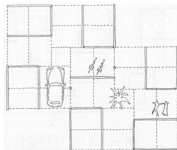
Abb. 180 : Grundriss einer Baueinheit und mögliche Anordnungen mehrerer Baueinheiten
