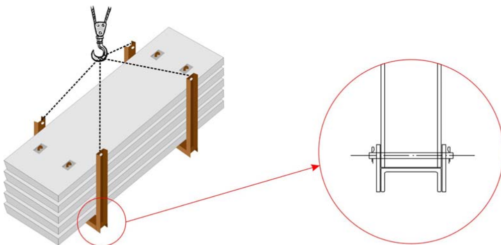
Abb. 87 : Zerlegbare Bündelrahmen
