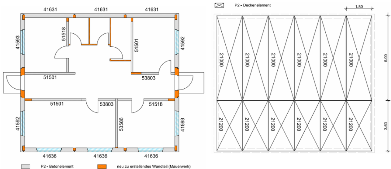
Abb. 175 : Entwurf eines Bürogebäudes Grundriss (li.) Deckenverlegeplan (re.)
