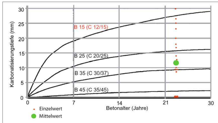
Abb. 45 : Karbonatisierungstiefe der Außenwände des Typs P2
