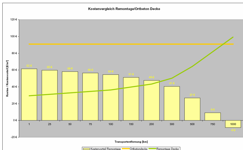
Abb. 120 : Vergleich der Deckenausführung in Ortbeton mit den Remontagekosten sekundärer Bauteile in Abhängigkeit der Transportentfernung (LKW) in Deutschland (beachte. verzerrte Darstellung der Transportentfernung)
