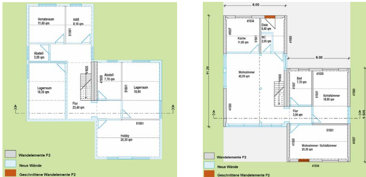
Abb. 140 : Grundrisse des Einfamilienhauses Kellergeschoss (li.), Erdgeschoss (re.)
