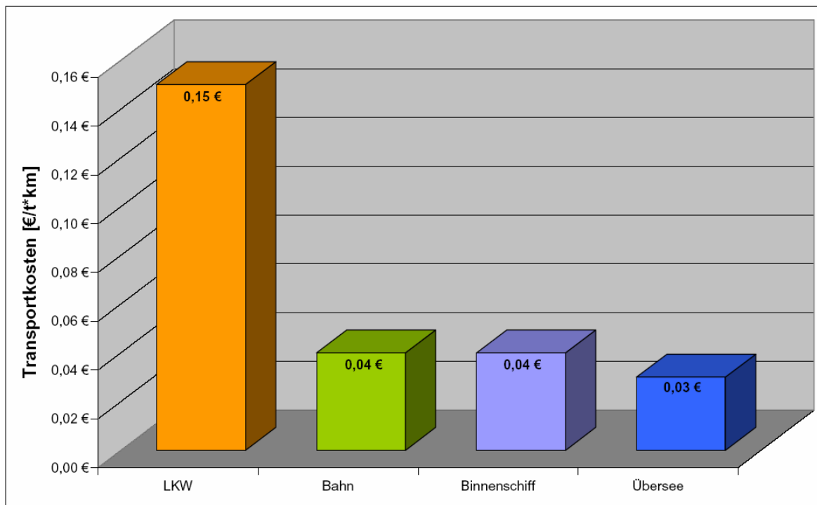
Abb. 107 : Abhängigkeit der Transportkosten von den Transportmitteln mit Bauteilumschlag
