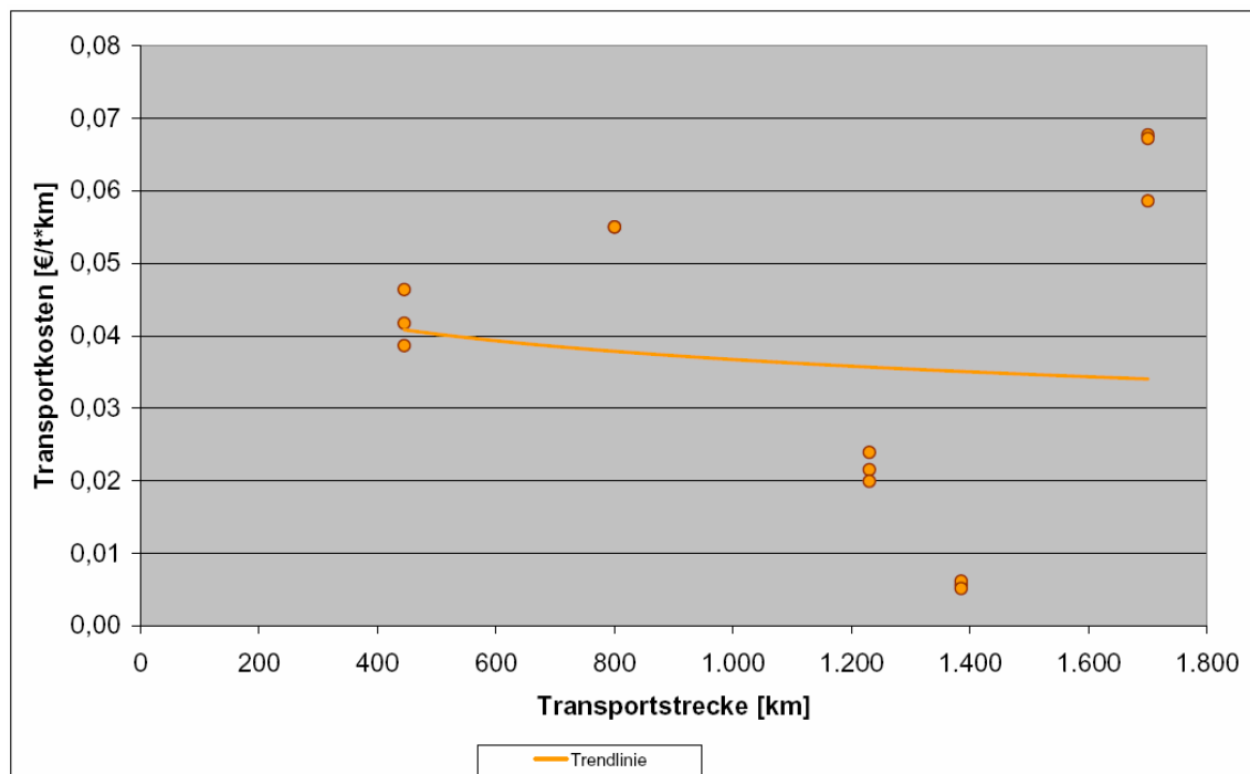
Abb. 104 : Abhängigkeit der Bahn-Transportkosten von der Transportentfernung
