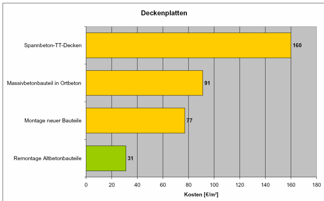
Abb. 113 : Vergleich der Remontagekosten mit den Kosten konventioneller Bauweisen zur Herstellung eines Quadratmeters Deckenfläche in Deutschland
