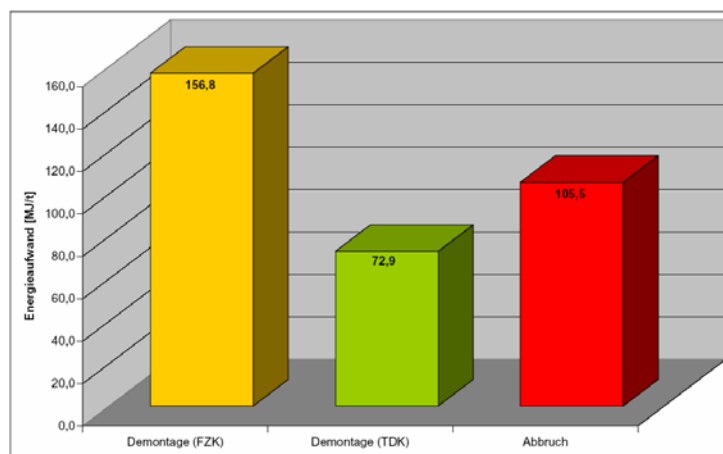
Abb. 128 : Vergleich der Energieaufwendungen für die Demontage und den Abbruch von einer Tonne Betonbauteile
