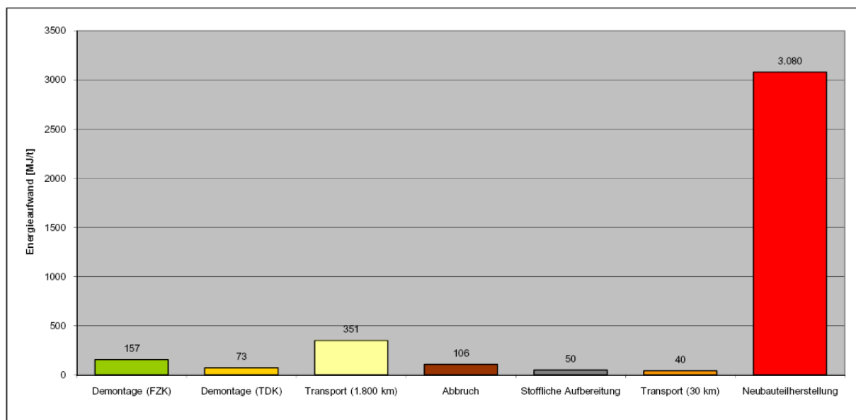
Abb. 130 : Grafische Darstellung der Zusammenstellung der ermittelten Energieaufwendungen für eine Tonne Betonbauteile
