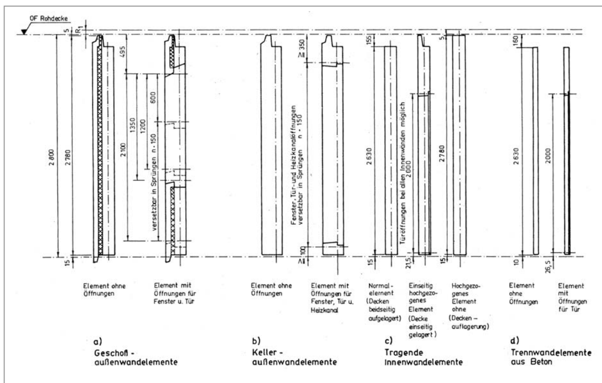
Abb. 31 : Auswahl an Wandelementen und Maßsystem 141
