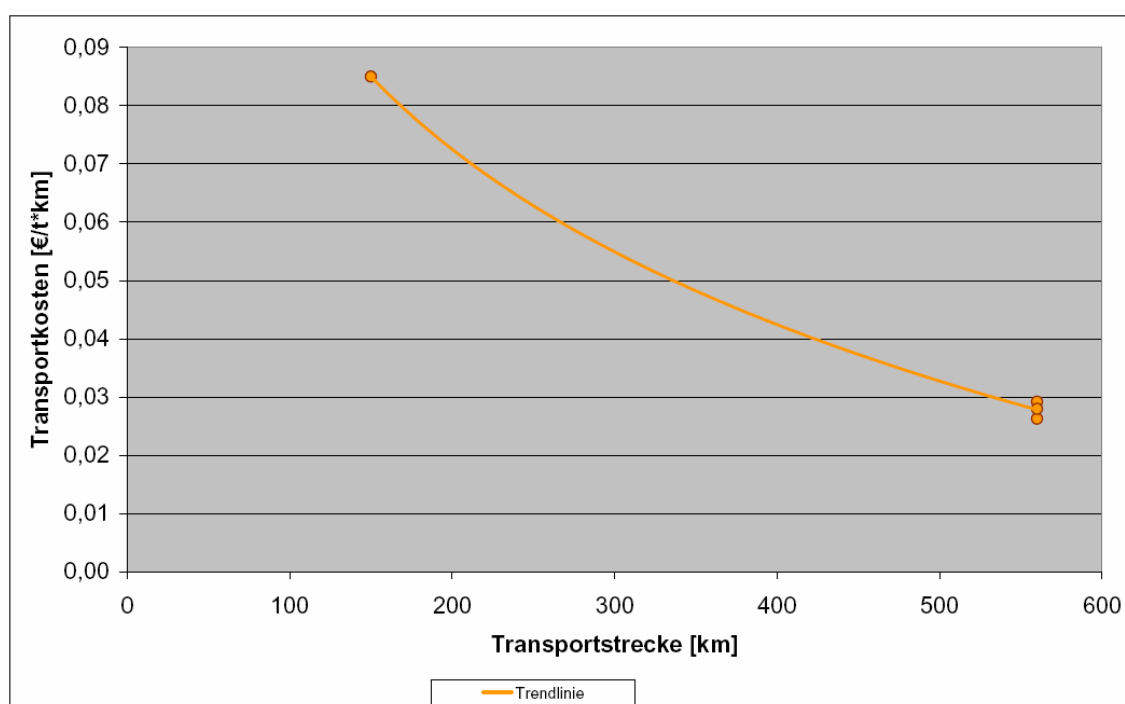
Abb. 105 : Abhängigkeit der Binnenschiff-Transportkosten von der Transportentfernung
