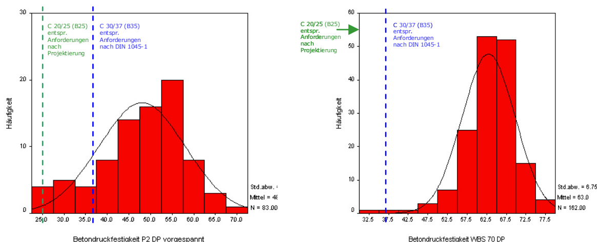
Abb. 36 : Häufigkeitsdiagramm ermittelter Druckfestigkeitswerte für Spannbetondeckenplatten P2 und WBS 70
