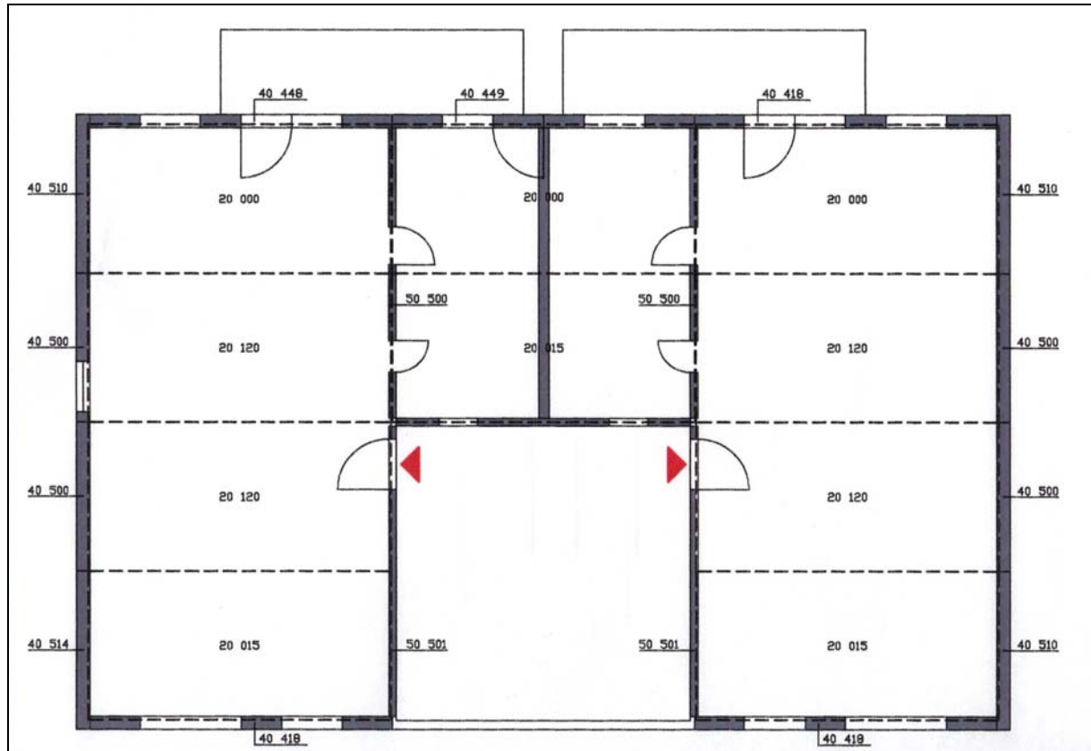
Abb. 144 : Grundriss des Musterhauses
