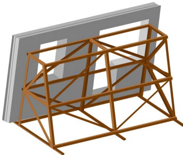
Abb. 88 : A-Bock
