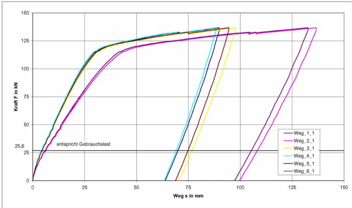
Abb. 64 : Kraft-Weg-Diagramm Stahlbetondecke 3, Elemente-Nr. 21 120
