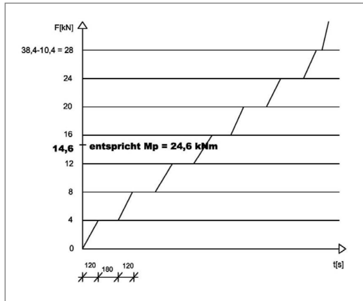
Abb. 57 : Last-Zeit-Diagramm, anlehnend an DIN EN 1356: 1997-2
