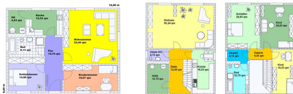
Abb. 153 : Grundriss der eingeschossigen Variante (98 m 2 ) (li.) sowie des Erd- (93 m 2 ) und Obergeschosses (84 m 2 ) der zweigeschossigen Variante – EFH 396
