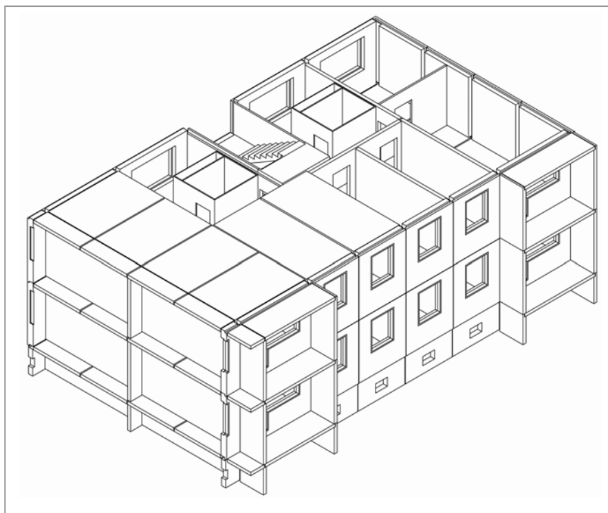
Abb. 16 : Räumliche Darstellung eines PN 36-NO-Segmentes (Rohbaumontage), Rückseite 98
