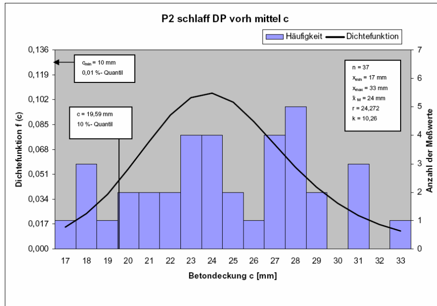
Abb. 50 : Graphische Darstellungen der Häufigkeitsverteilung der vorhandenen mittleren Betondeckung c von 37 schlaff bewehrten Deckenplatten der Typenserie P2
