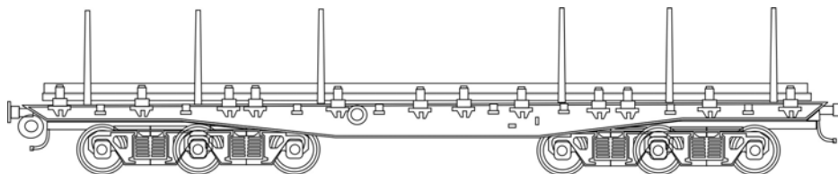
Abb. 82 : Drehgestellflachwagen mit sechs Radsätzen der Güterwagengattungen S 268
