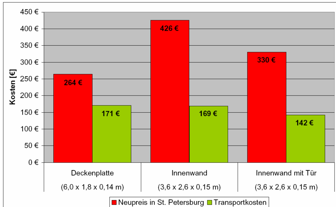
Abb. 111 : Vergleich der Preise für Betonelemente hergestellt in St. Petersburg und den Transportkosten für sekundäre Betonbauteile aus Deutschland (ohne Bereitstellungs- und Prüfkosten)
