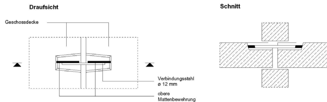
Abb. 26 : Verbindung Decke – Decke, längs zur Spannrichtung 126
