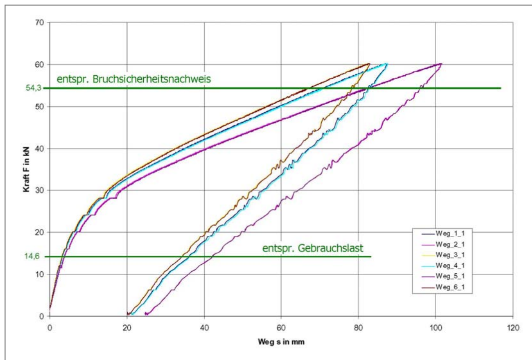
Abb. 58 : Kraft-Weg-Diagramm Spannbetondeckenplatte 1, Elemente-Nr. 22006
