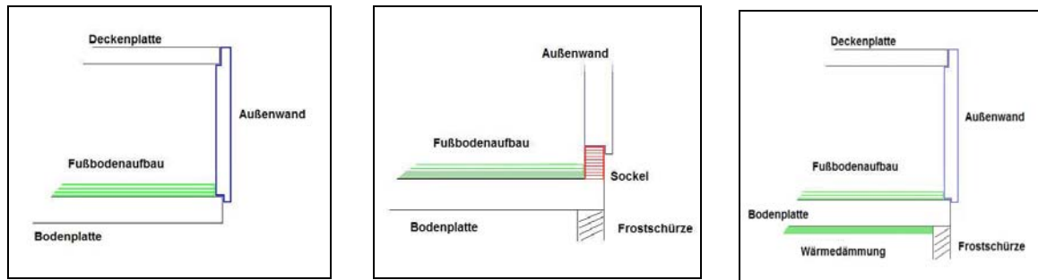
Abb. 145 : Alternativen zur Gestaltung der Raumhöhe durch Fußbodenaufbau, Sockel, Wärmedämmung (v.l.n.r.)
