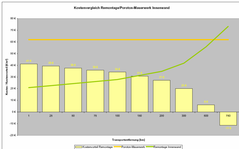
Abb. 119 : Vergleich der Innenwandausführung in Poroton-Mauerwerk mit den Remontagekosten sekundärer Bauteile in Abhängigkeit der Transportentfernung (LKW) in Deutschland (beachte. verzerrte Darstellung der Transportentfernung)
