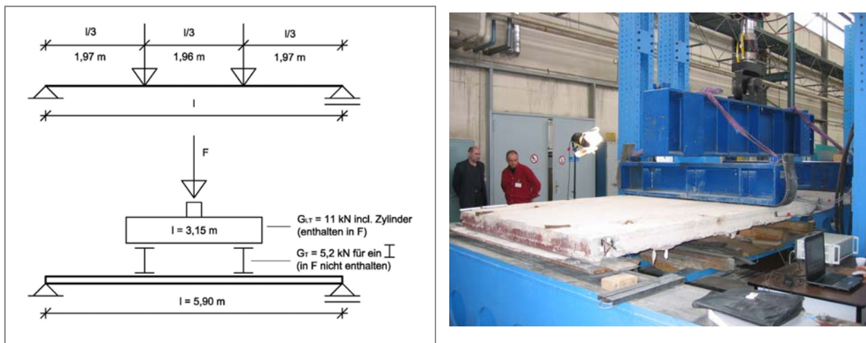
Abb. 54 : Belastungsanordnung und Einrichtung Spannbetondeckenplatte 22 006 (li.) und Versuchseinrichtung (re.)
