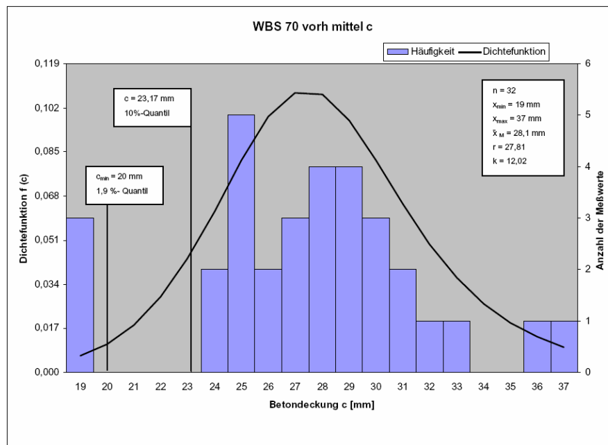
Abb. 48 : Graphische Darstellung der Häufigkeitsverteilung der vorhandenen mittleren Betondeckung c von 32 Spannbetondeckenplatten des Typs WBS 70
