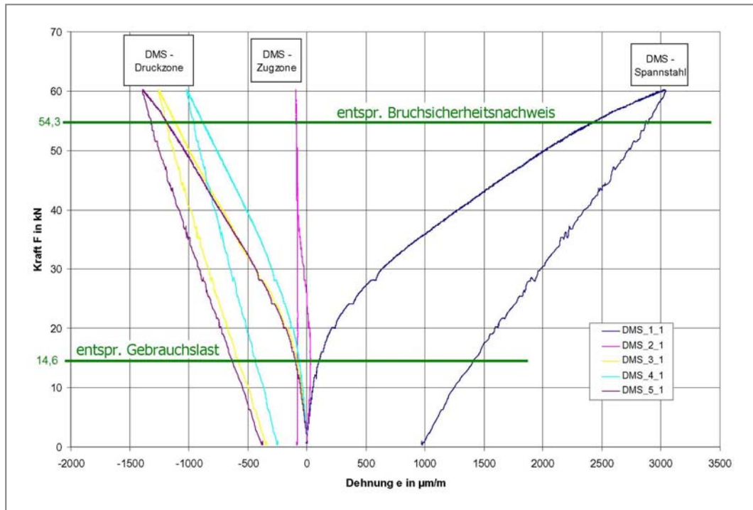
Abb. 59 : Kraft-Dehnungs-Diagramm Spannbetondecke 1, Elemente-Nr. 22006
