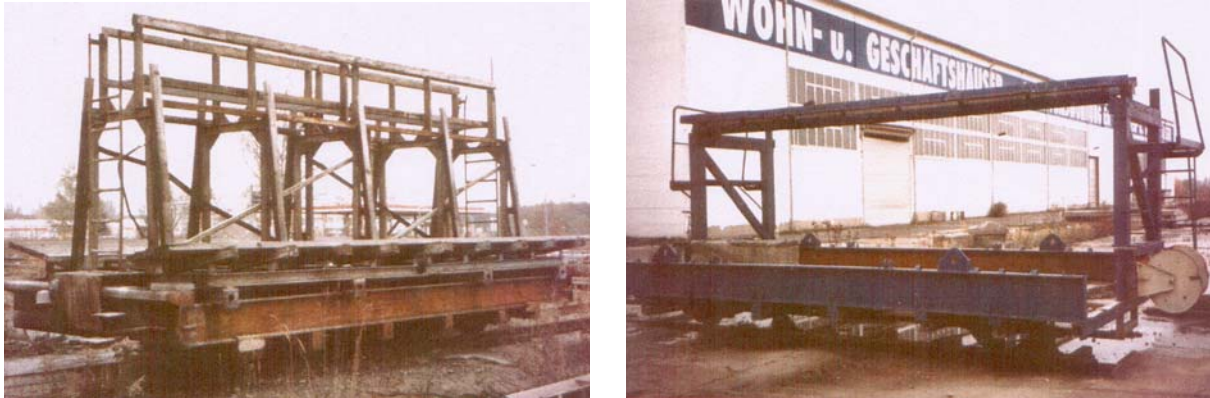
Abb. 89 : Ausfahrpaletten im Betonwerk Hoyerswerda 288
