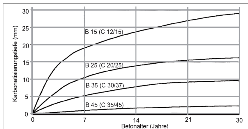
Abb. 38 : Entwicklung der Karbonatisierungstiefe in Abhängigkeit von der Festigkeitsklasse und der Zeit 182
