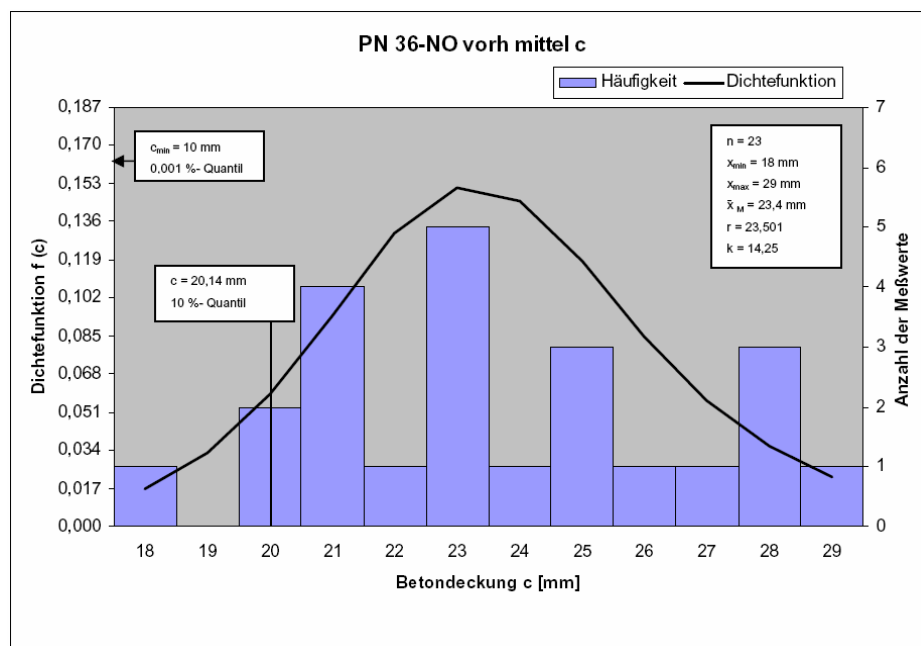
Abb. 52 : Graphische Darstellung der Häufigkeitsverteilung der vorhandenen mittleren Betondeckung c von 23 Geschloßdecken des Bautyps PN 36-NO
