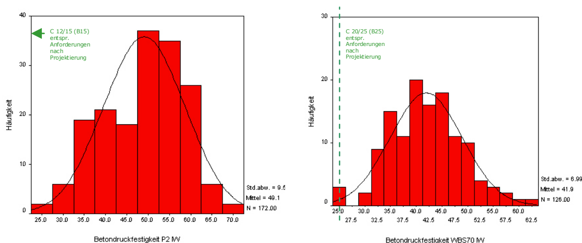
Abb. 37 : Häufigkeitsdiagramm ermittelter Druckfestigkeitswerte für Innenwandelemente P2 und WBS 70
