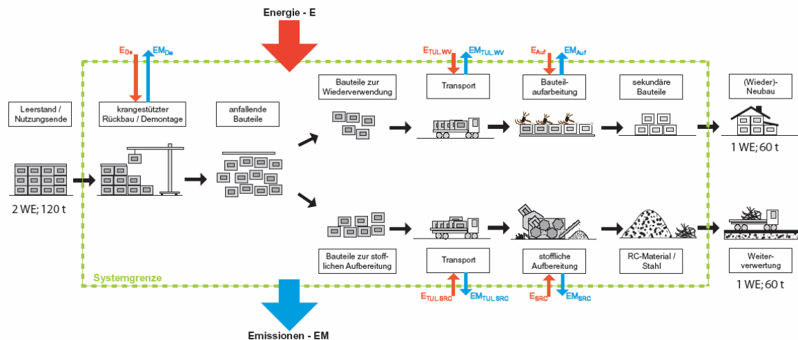
Abb. 126 : Systemgrenzen des Öko-Screenings Szenario 1
