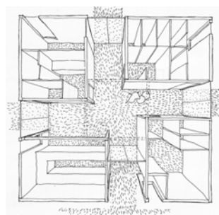
Abb. 181 : Entwurf einer Raststätte aus einer Baueinheit als quadratische Variante, mehreren Baueinheiten als Längsvariante
