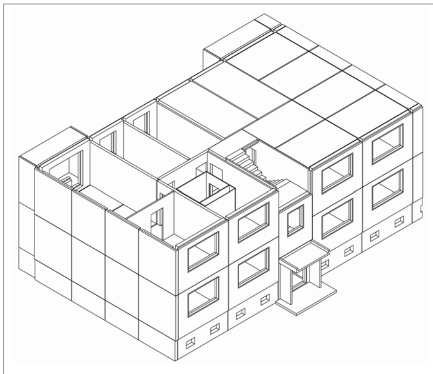
Abb. 15 : Räumliche Darstellung eines PN 36-NO-Segmentes (Rohbaumontage), Eingangsseite 97
