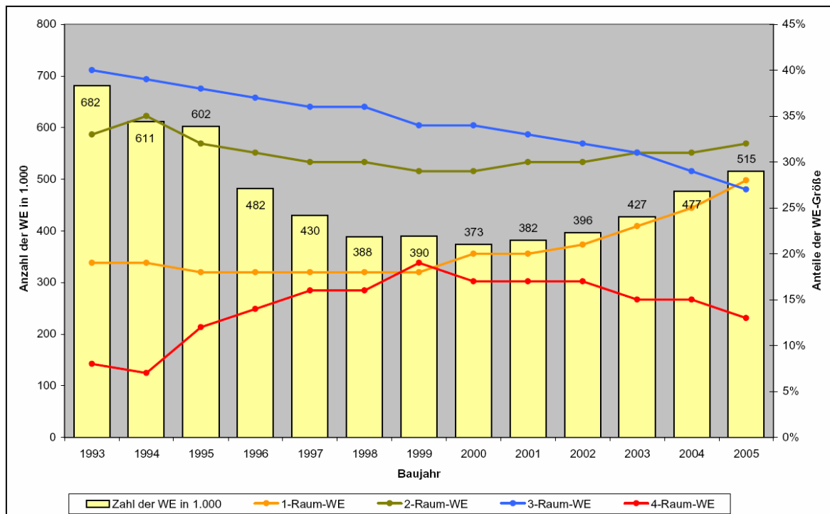
Abb. 8 : Anzahl der neu gebauten Wohnungen in Russland (in 1.000) und deren Anteile entsprechend der durchschnittlichen Größe) 65
