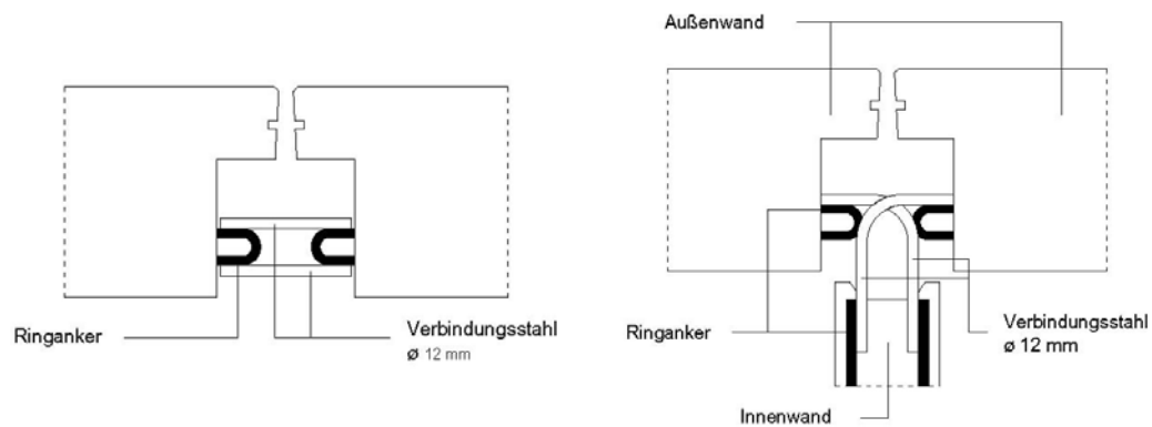
Abb. 24 : Ringankerbewehrung und Verbindung Außenwände - Innenwände 124
