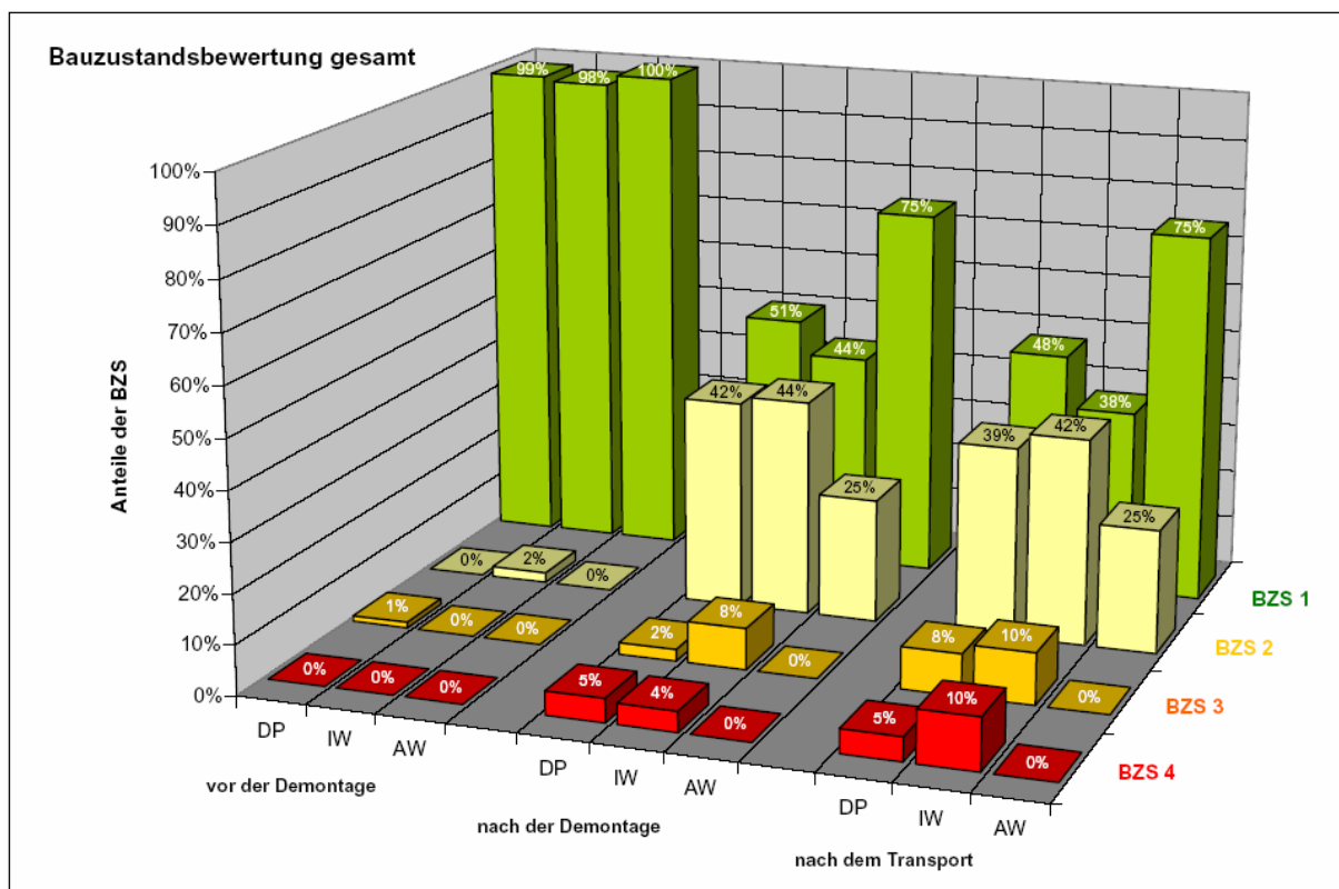
Abb. 79 : Zusammenstellung der Ergebnisse der Bauzustandsuntersuchungen über den gesamten Rückbauprozess (Fallbeispiel Gröditz)
