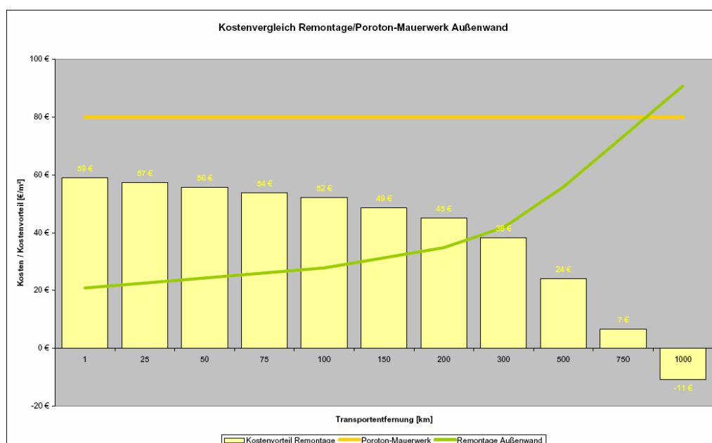
Abb. 118 : Vergleich der Außenwandausführung in Poroton-Mauerwerk mit den Remontagekosten sekundärer Bauteile in Abhängigkeit der Transportentfernung (LKW) in Deutschland (beachte. verzerrte Darstellung der Transportentfernung)
