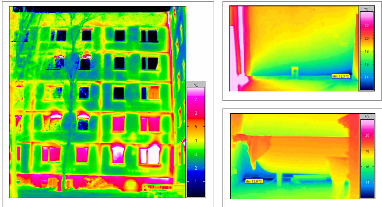
Abb. 66 : Infrarotaufnahmen einer Gebäuderückseite (li.); Anschluss Giebelaußenwand-Kellerdecke EG im Kinderzimmer (re. oben), im Bad (re. unten)
