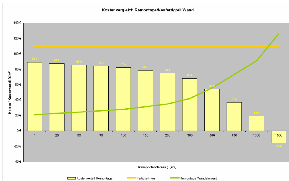
Abb. 116 : Vergleich der Kosten für die Montage von neuen Wandelementen mit den Remontagekosten sekundärer Bauteile in Abhängigkeit der Transportentfernung (LKW) in Deutschland (beachte. verzerrte Darstellung der Transportentfernung)
