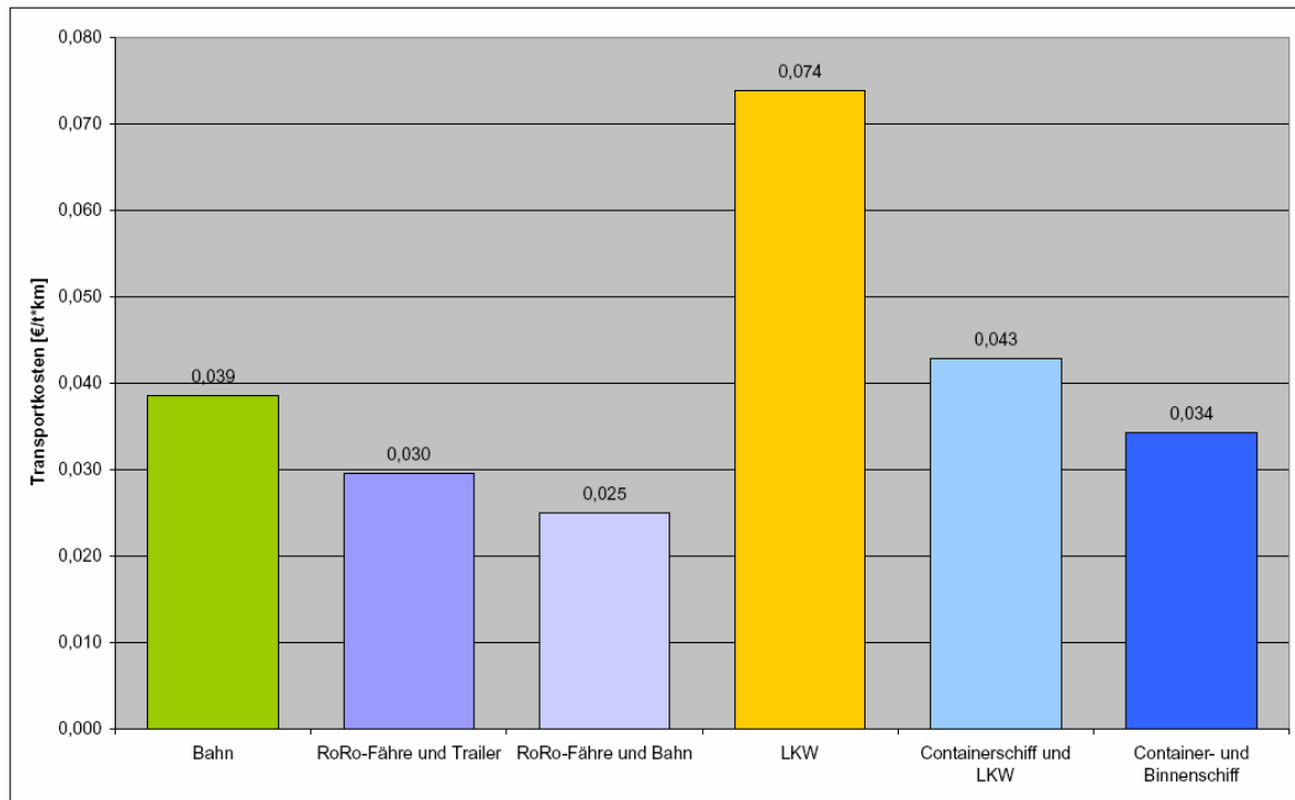
Abb. 108 : Vergleich der Kosten der verschiedenen Transportkombinationen
