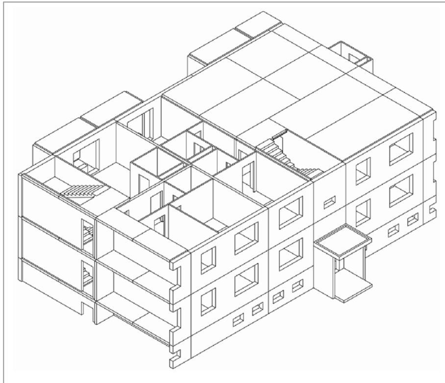
Abb. 27 : Prinzipdarstellung eines Segments der Typenserie WBS 70 6,3t (Standort Templin) 132
