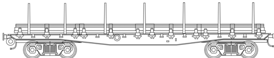
Abb. 81 : Drehgestellflachwagen mit vier Radsätzen der Güterwagengattung R 266
