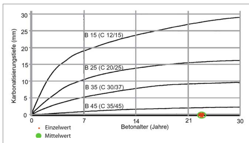
Abb. 43 : Darstellung der Karbonatisierungstiefe der Deckenplatten des Typs P2
