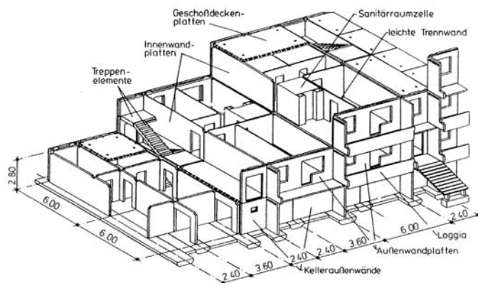
Abb. 28 : Räumliche Prinzipdarstellung der WBS 70-Montagebauweise 133
