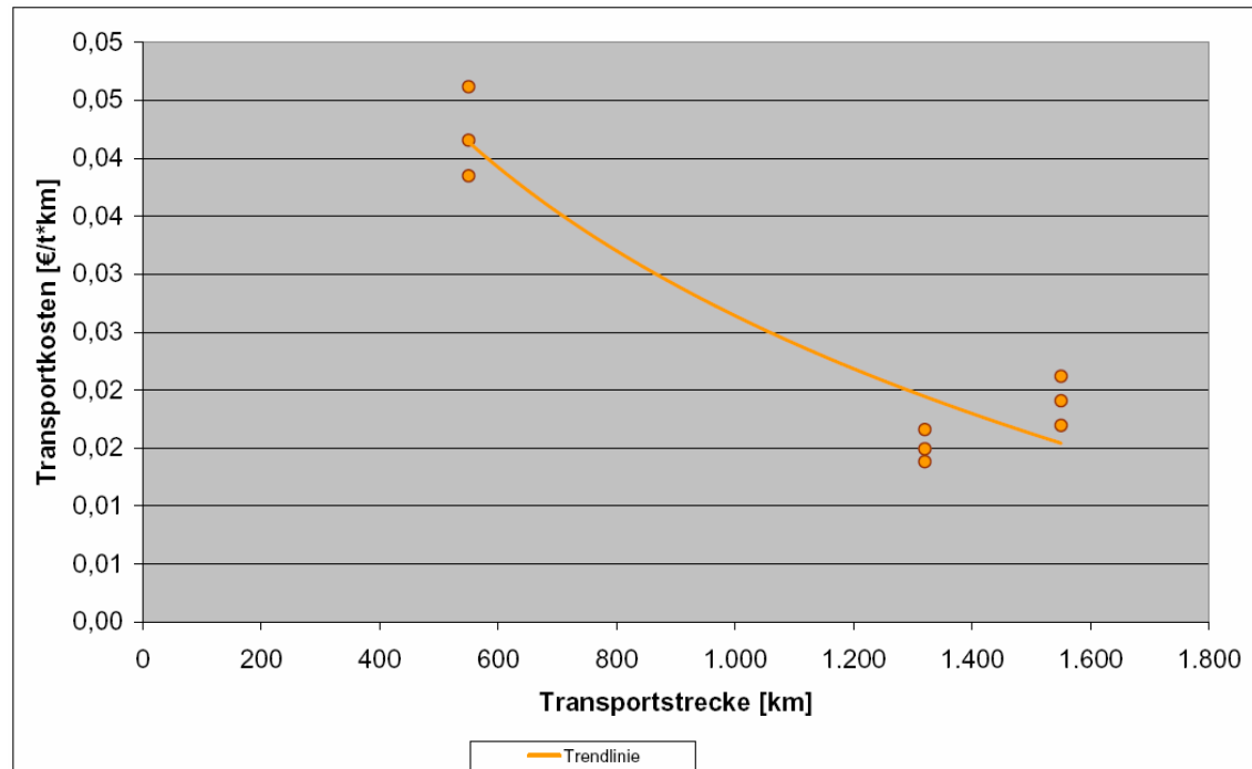
Abb. 106 : Abhängigkeit der See-Transportkosten von der Transportentfernung
