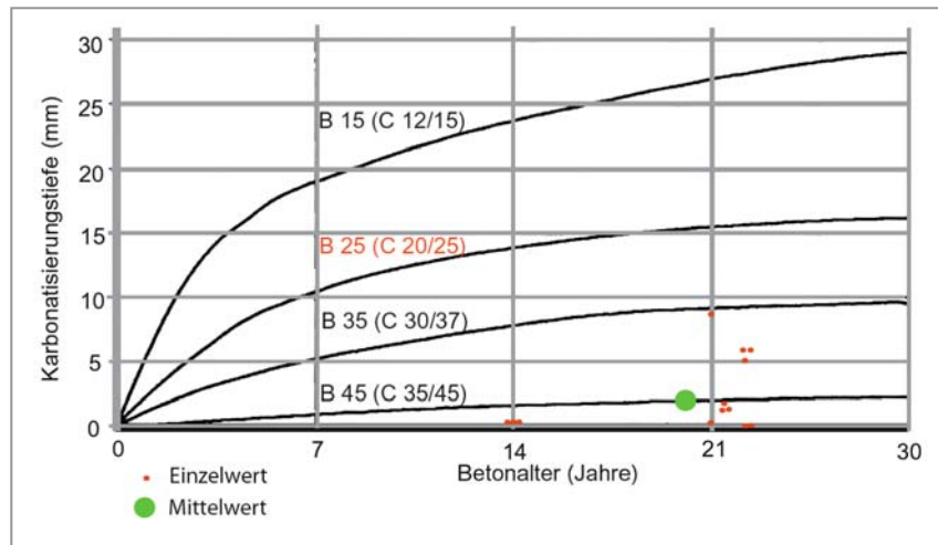
Abb. 41 : Karbonatisierungstiefe der Innenwände des Typs WBS 70
