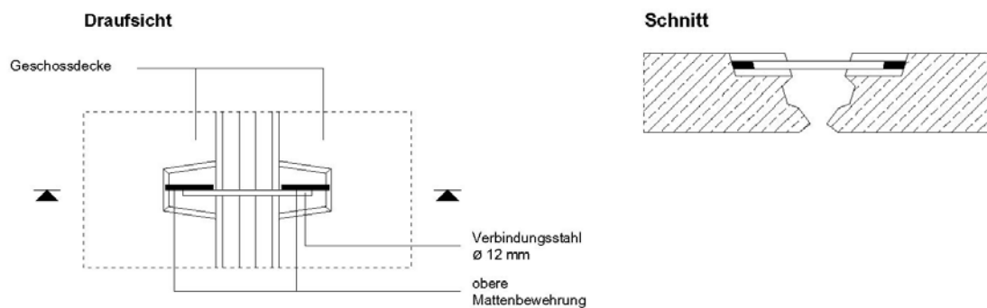
Abb. 25 : Verbindung Decke – Decke, quer zur Spannrichtung 125
