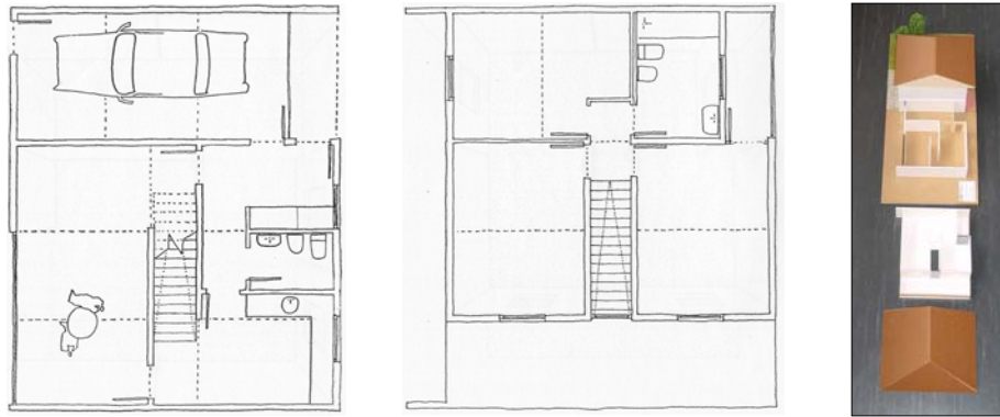
Abb. 148 : Grundrisse der Doppelhaus-Konstruktion
