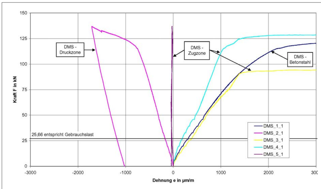
Abb. 65 : Kraft-Dehnungs-Diagramm Stahlbetondecke 3, Elemente-Nr. 21 120
