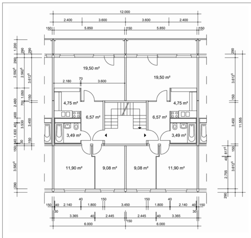
Abb. 21 : Grundriss Normalgeschoss – Segment der Plattenbauserie P2 (5,0 t) 110
