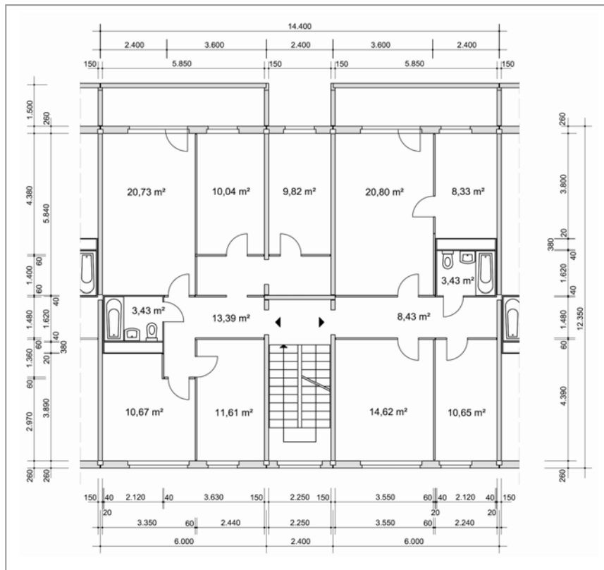
Abb. 30 : Segmentgrundriss eines WBS 70-Wohngebäudes 134
