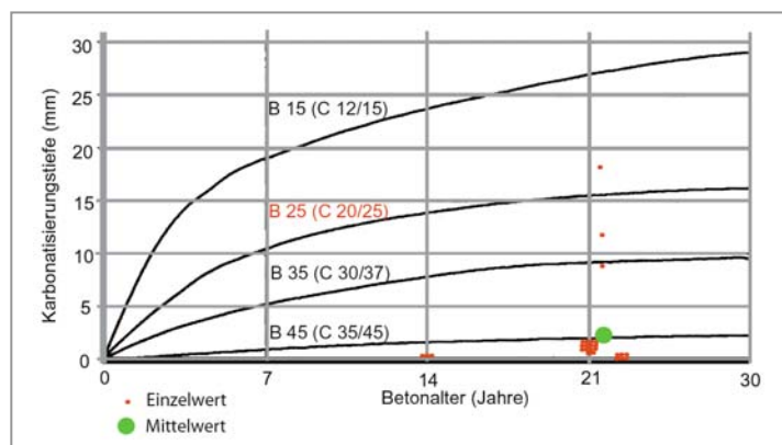
Abb. 40 : Darstellung der Karbonatisierungstiefe der Deckenplatten des Typs WBS 70
