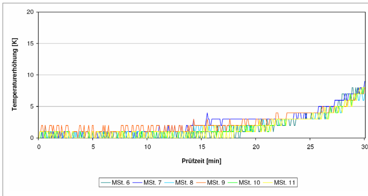
Abb. 73 : Temperaturerhöhung auf der unbeflammten Deckenoberfläche – Spannbetondeckenplatte 21000 (Probe I)
