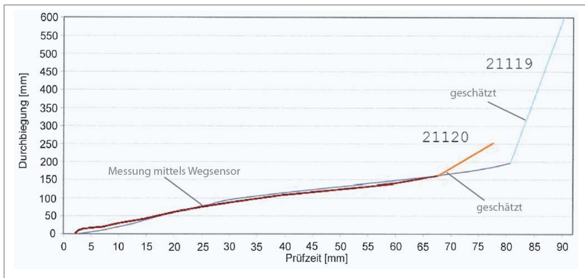
Abb. 75 : Durchbiegung in Richtung Brandraum – Stahlbetondeckenplatten 21119, 21120 (P2-Typ)
