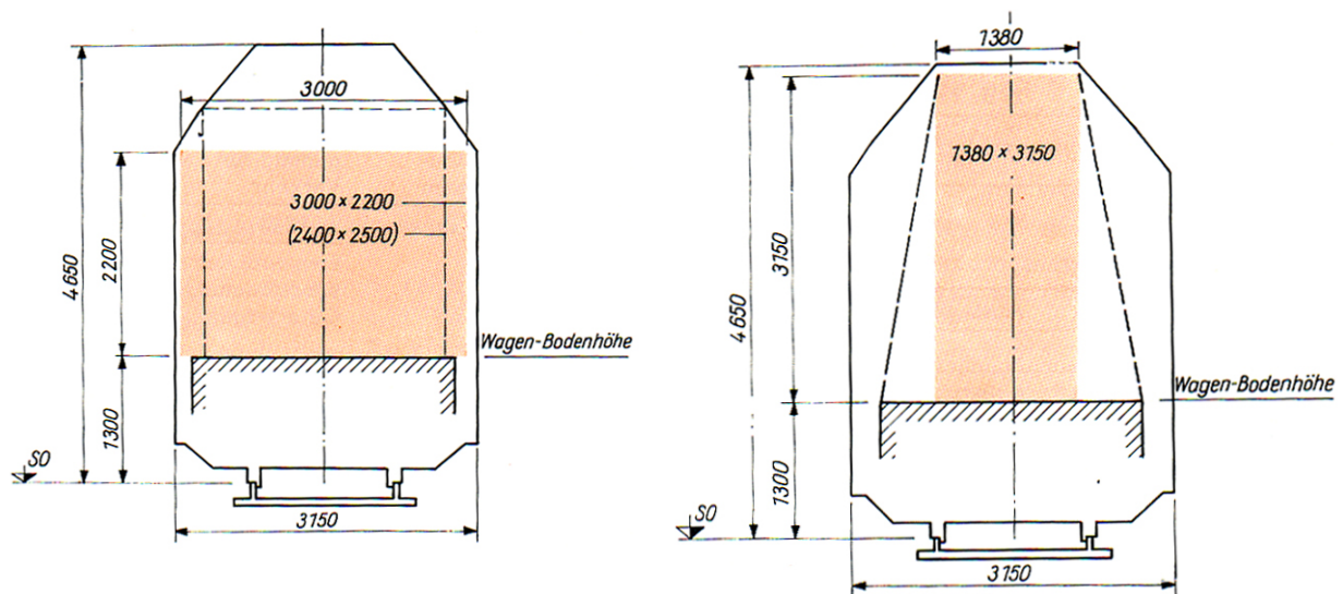
Abb. 83 : Ladeprofil für den liegenden und stehenden Transport von Betonfertigteilen 273
