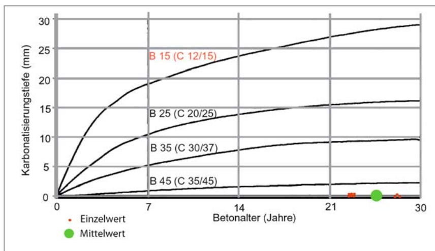
Abb. 44 : Darstellung der Karbonatisierungstiefe der Innenwände des Typs P2
