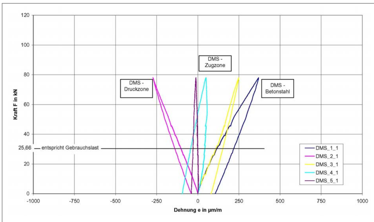
Abb. 63 : Kraft-Dehnungs-Diagramm Stahlbetondecke 2, Elemente-Nr. 21 120
