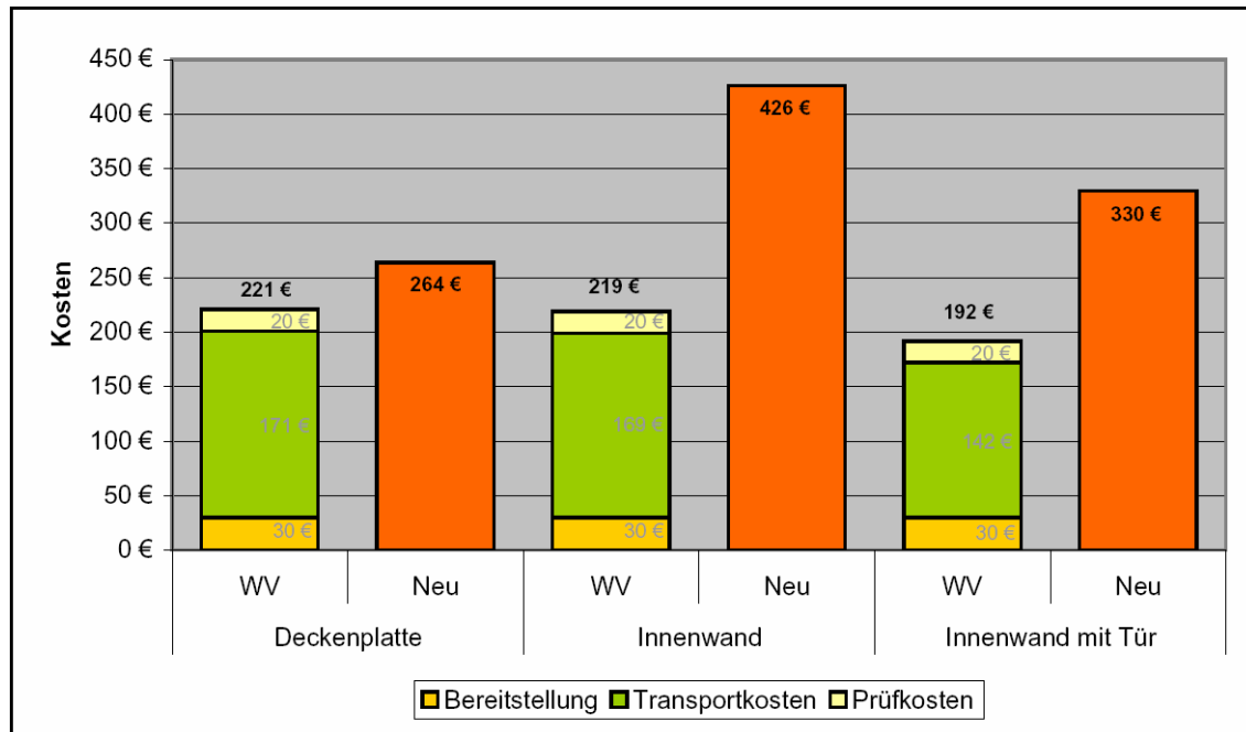
Abb. 112 : Vergleich der Preise für Betonelemente hergestellt in St. Petersburg und den Kosten für den Einsatz sekundärer Betonbauteile aus Deutschland (mit Bereitstellungs- und Prüfkosten)
