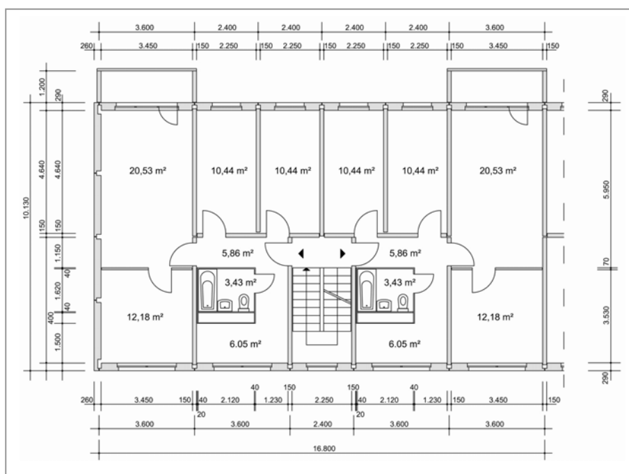
Abb. 17 : Normalgeschossgrundriss eines 16,80 m breiten PN 36-NO-Segmentes 99
