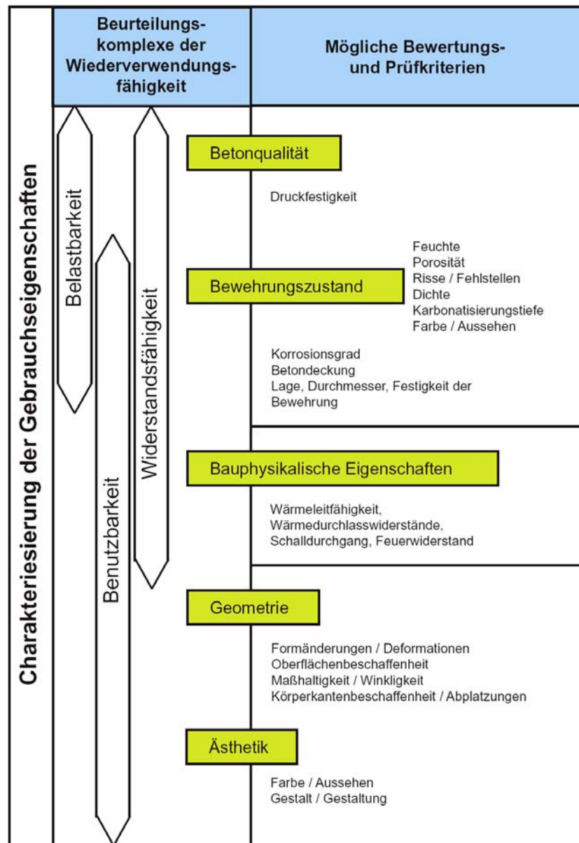
Abb. 35 : Untersuchungsprogramm Bauzustand Betonelemente 158
