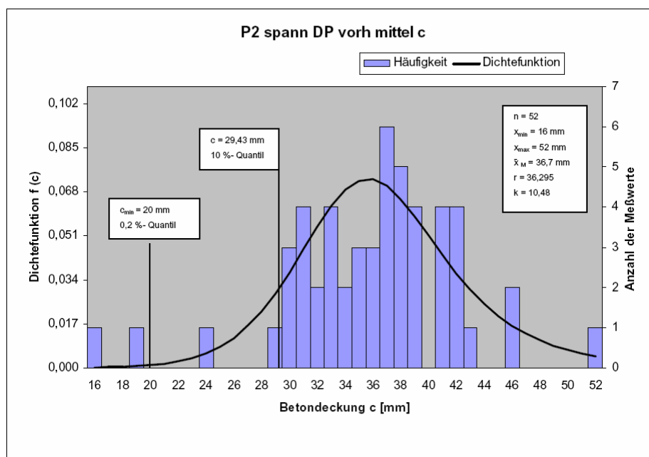
Abb. 49 : Graphische Darstellung der Häufigkeitsverteilung der vorhandenen mittleren Betondeckung c von 52 Spannbetondeckenplatten des Typs P2
